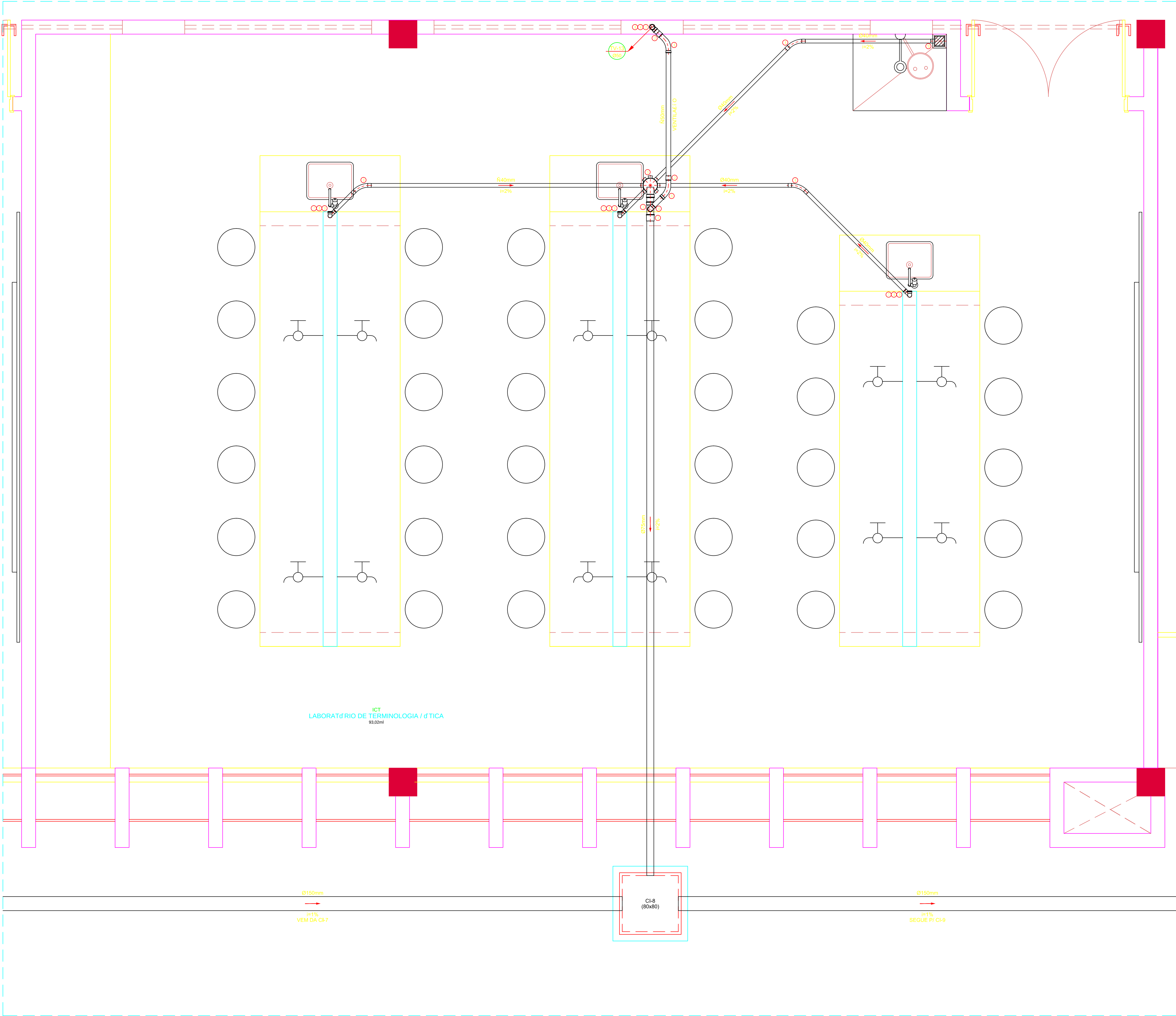
DETALHE 6 ESCALA: 1/20
