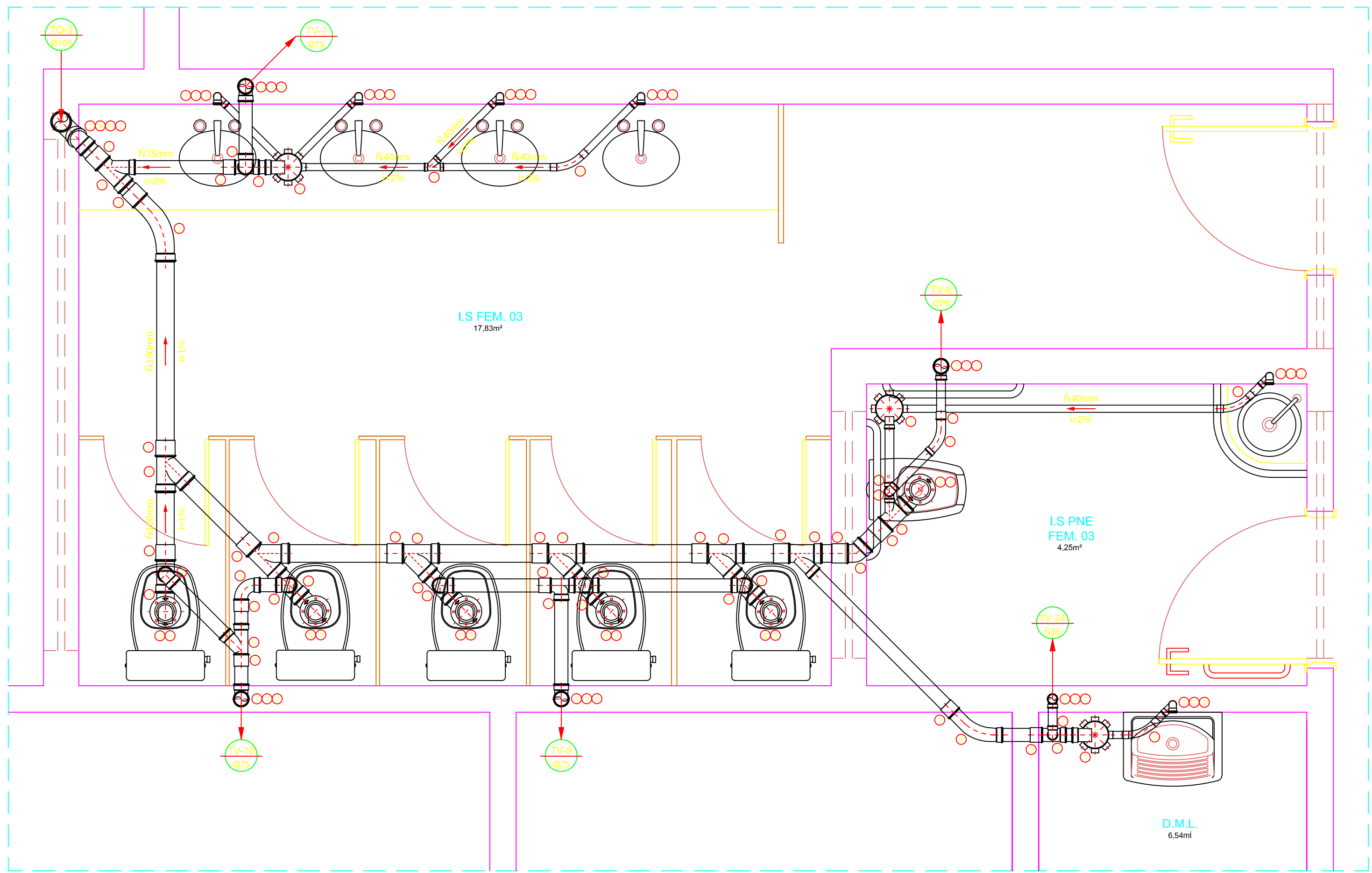
DETALHE 12-14 ESCALA: 1/20
