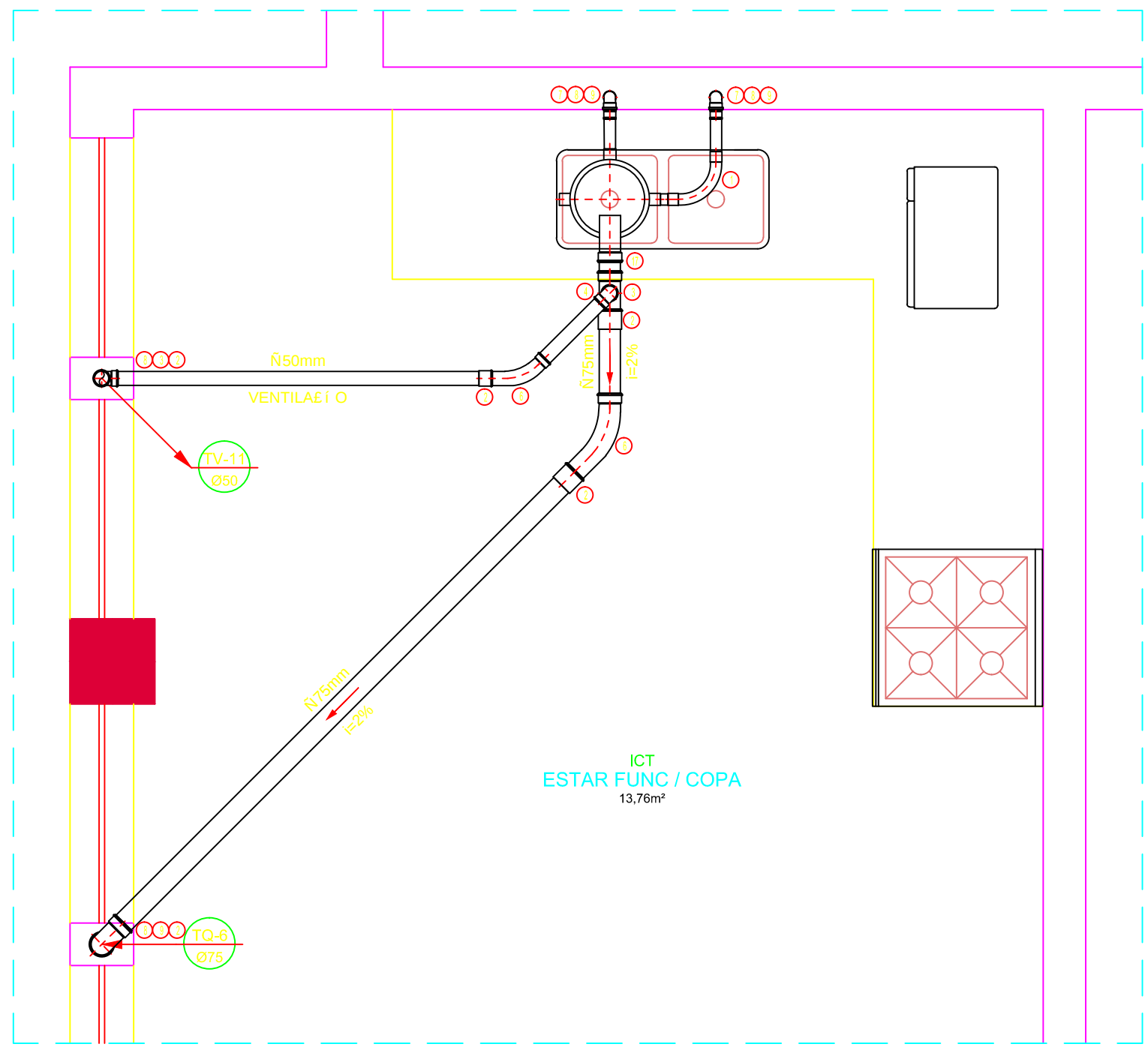
DETALHE 13 ESCALA: 1/20
