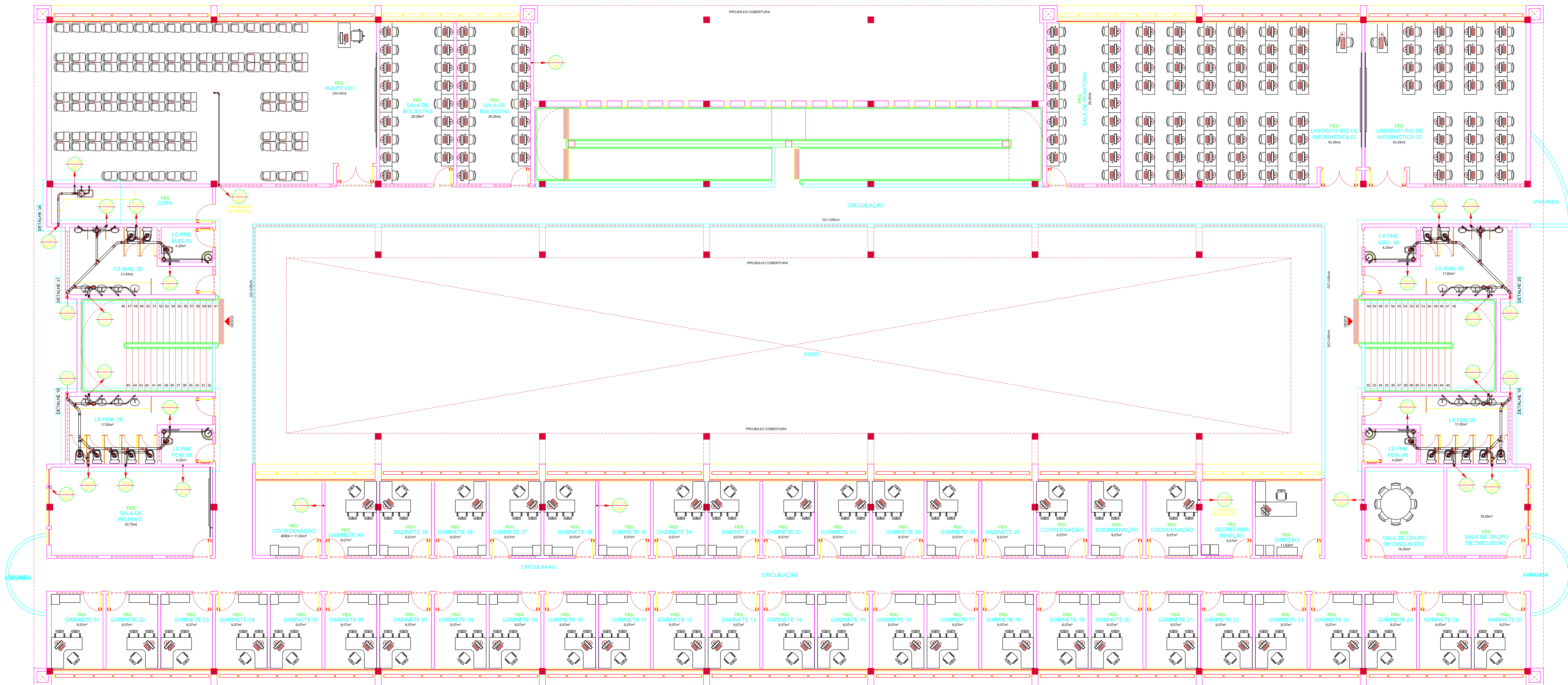
PLANTA BAIXA - 3ºPISO ESCALA: 1/75 - CREA: 1.839,04m
