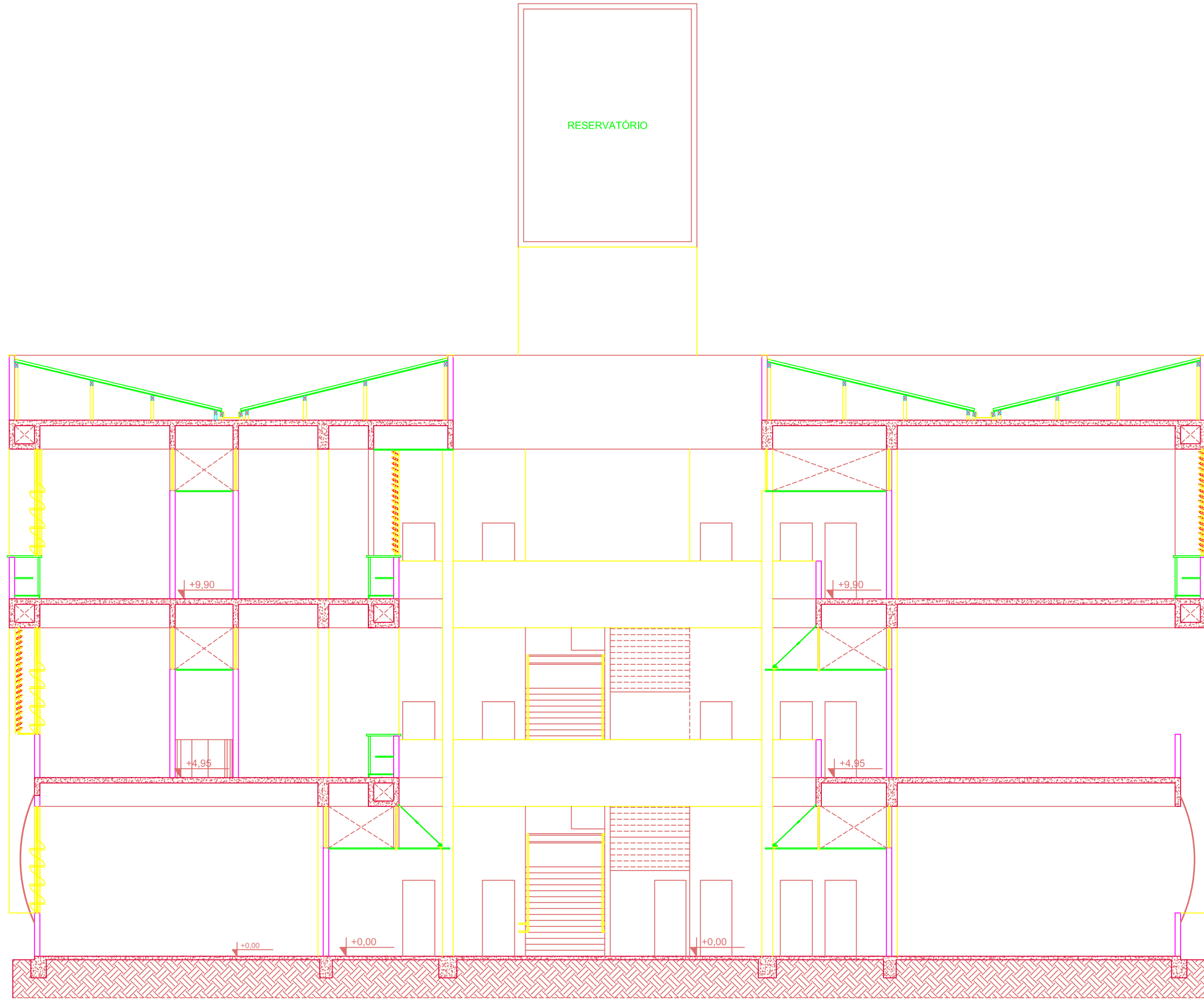
CORTE C1 ESCALA: 1/100
