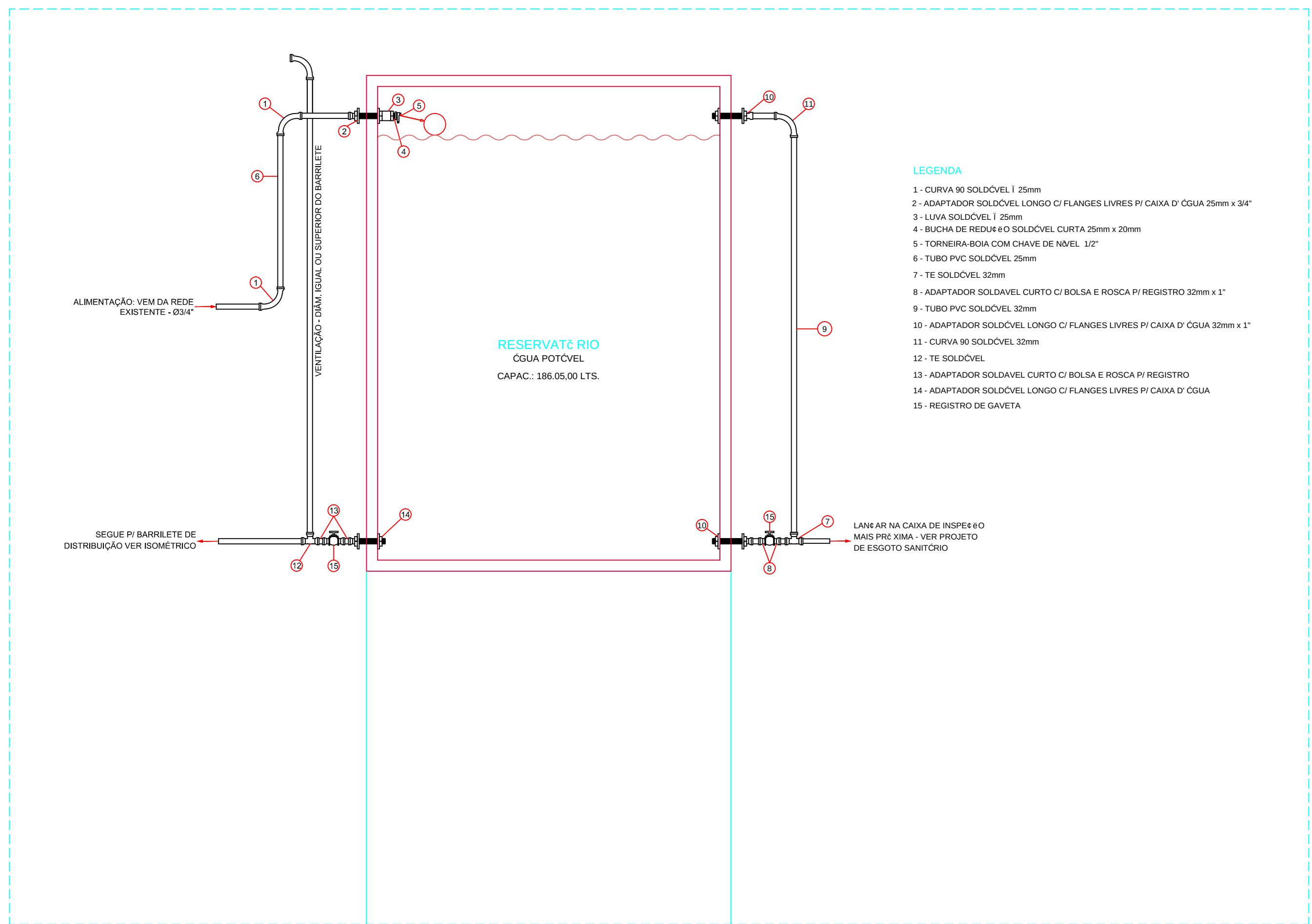
DETALHE ESQUEMÁTICO DA INSTALAÇÃO DO RESERVATÓRIO SUPERIOR SEM ESCALA
