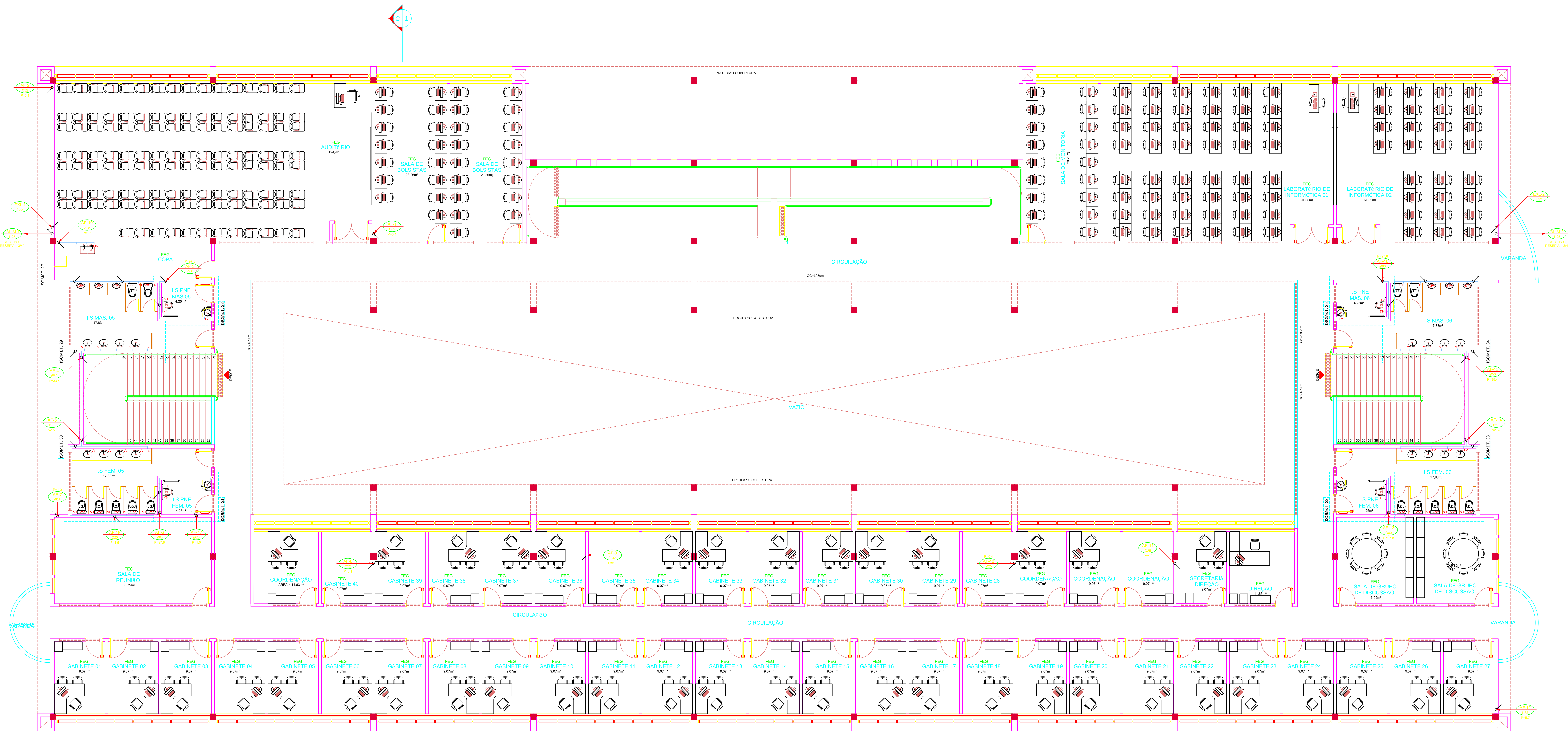
PLANTA BAIXA - 3º FLO ESCALA: 1/75 - CREA: 1.839,04m
