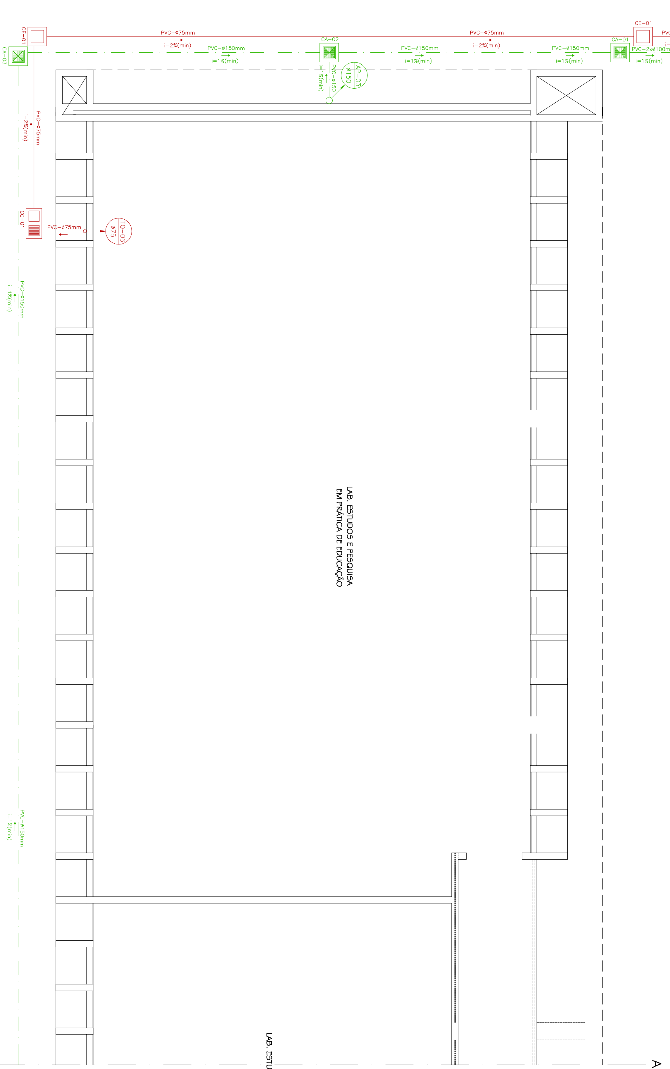
Planta Baixa - 1º Pavimento Projeto Sanitário e Águas Pluviais ESC: 1:50
