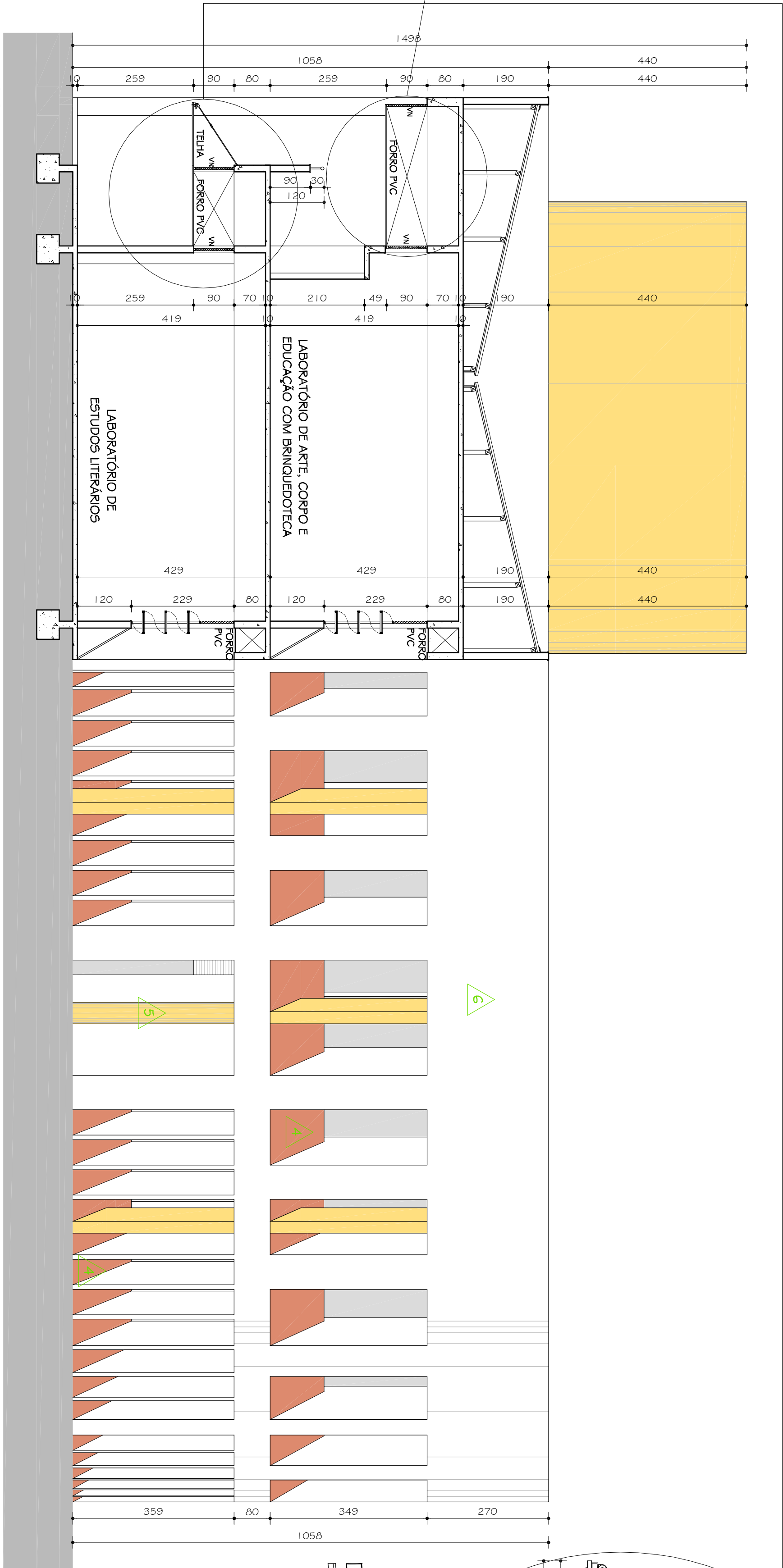
DETALHE 02 Esc. 1:25
