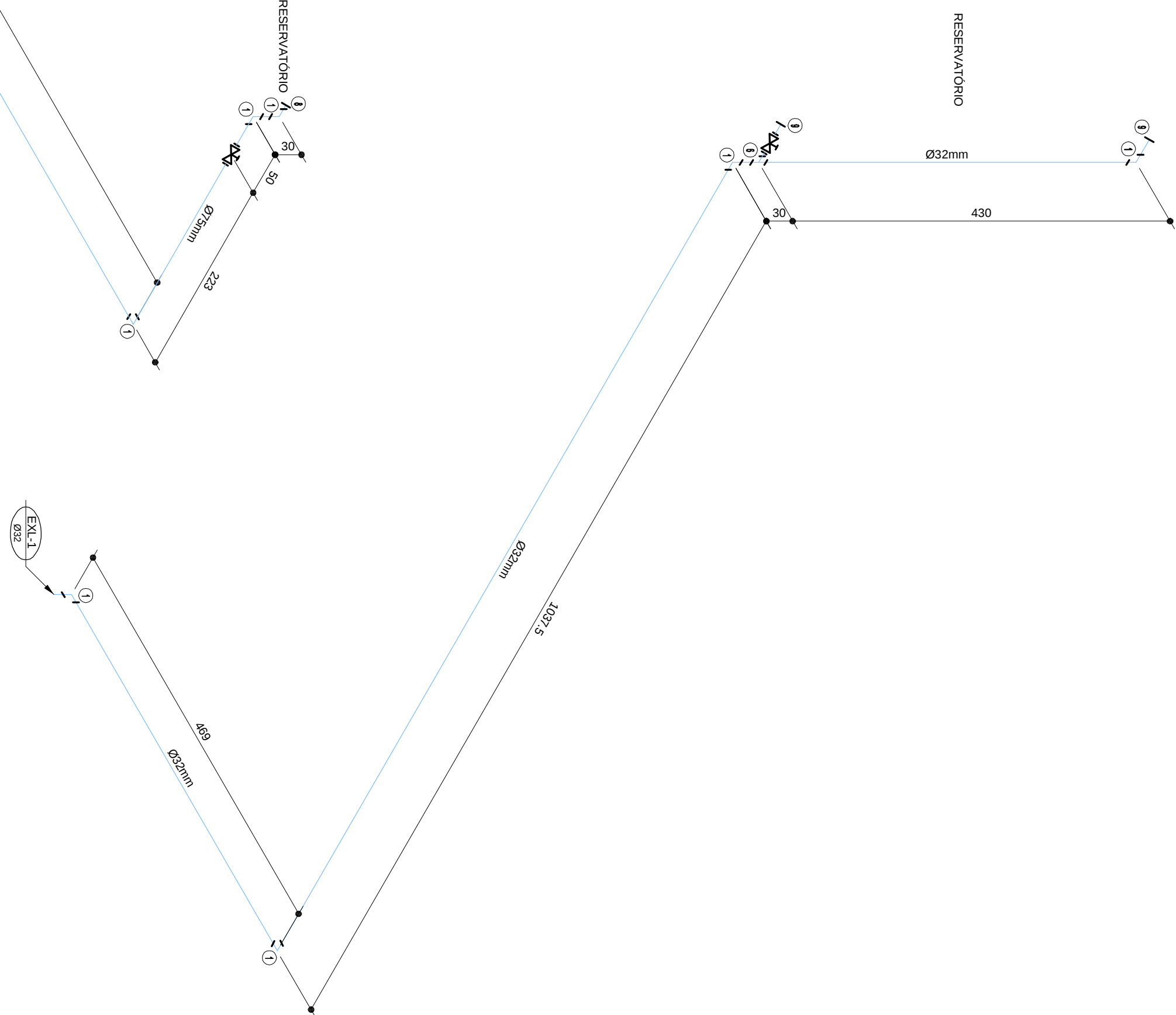
ISOMÉTRICO - EXTRAVASSOR E LIMPEZA Esc. 1:50
