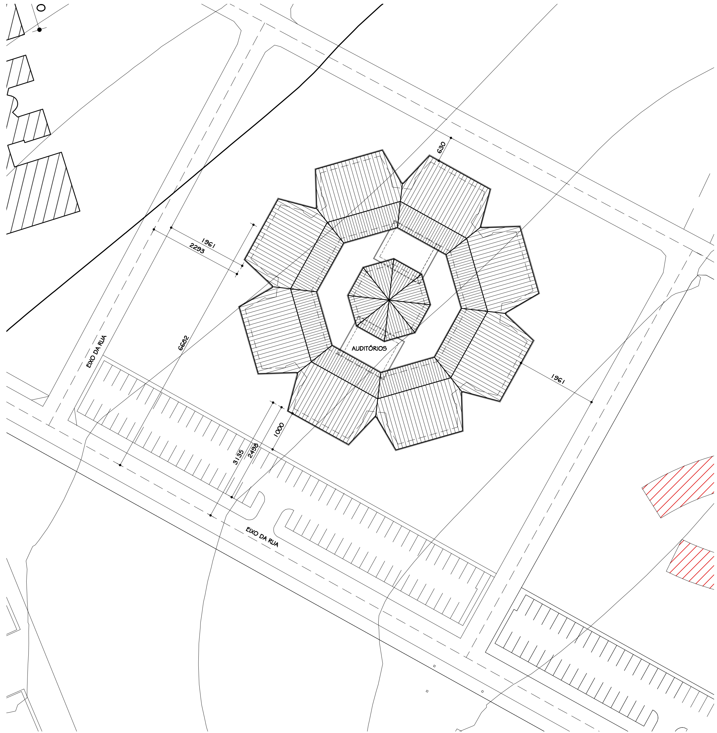
PLANTA LOCAÇÃO PRÉDIO SALAS AUDITÓRIO ESC. 1:500
