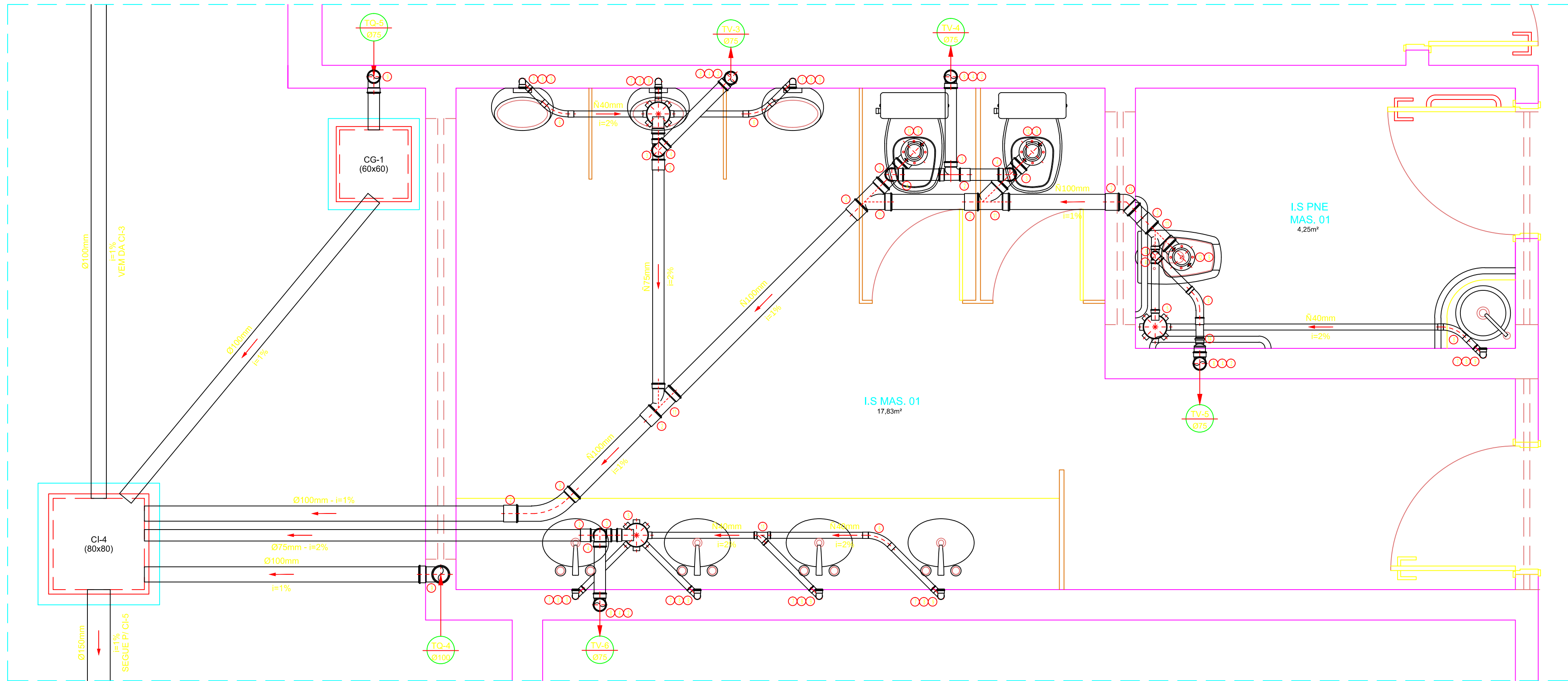
DETALHE 3=10 ESCALA: 1/20
