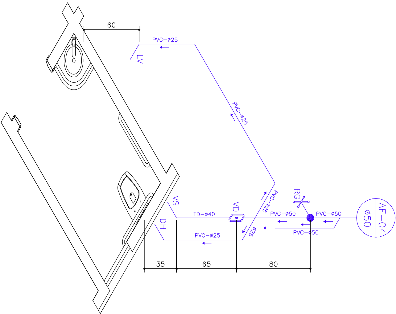
Isométrico 04: I.S. PNE Feminino Água Fria - Pavto Tipo Esc: 1:25
