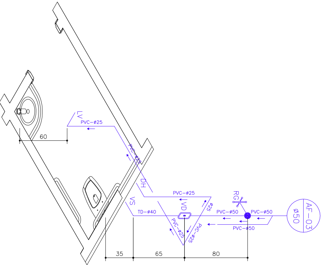
Isométrico 03: I.S. PNE Masculino Água Fria - Pavto Tipo Esc: 1:25
