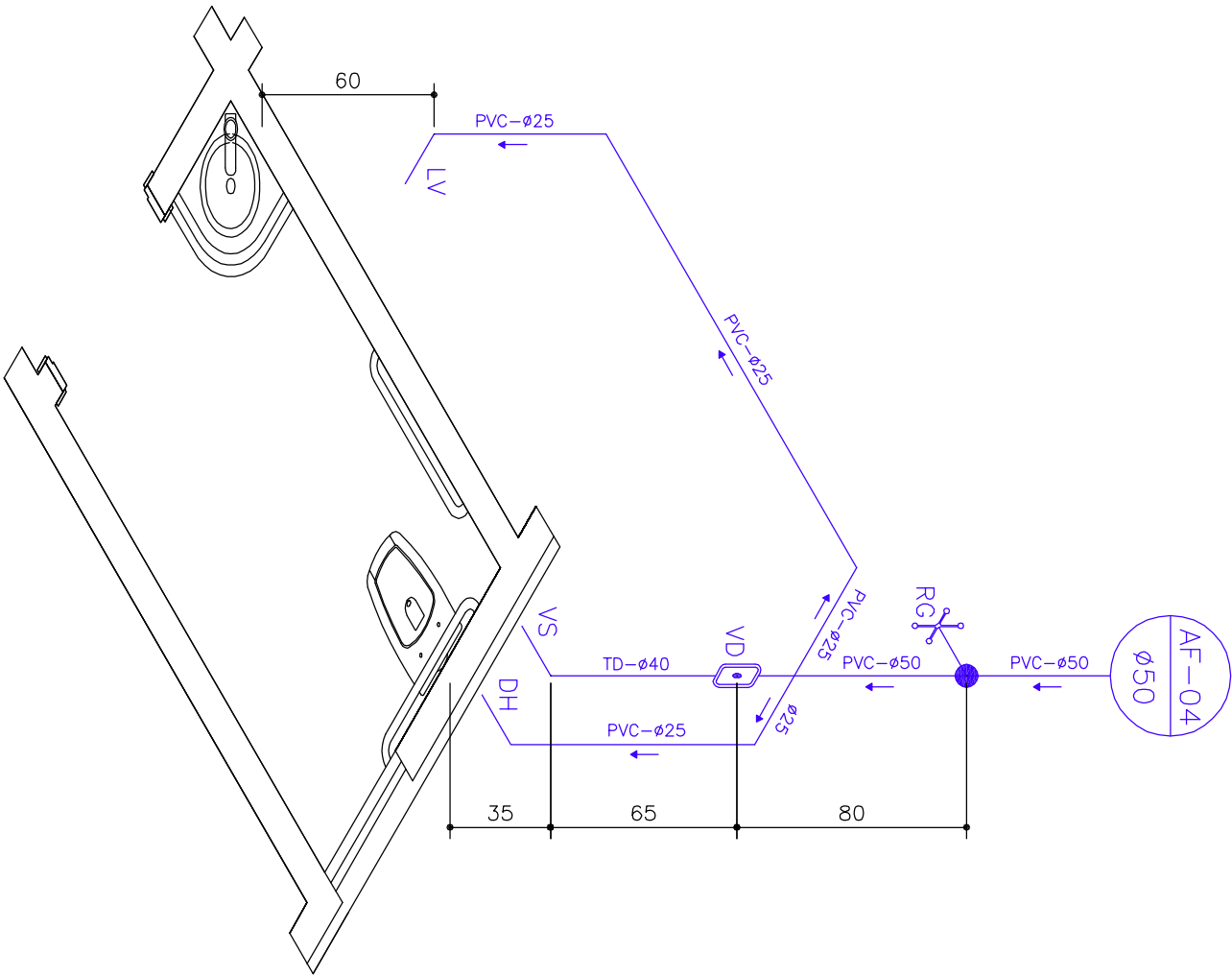
Isométrico 04: I.S. PNE Feminino Água Fria - Pavão Térreo Esc: 1:25
