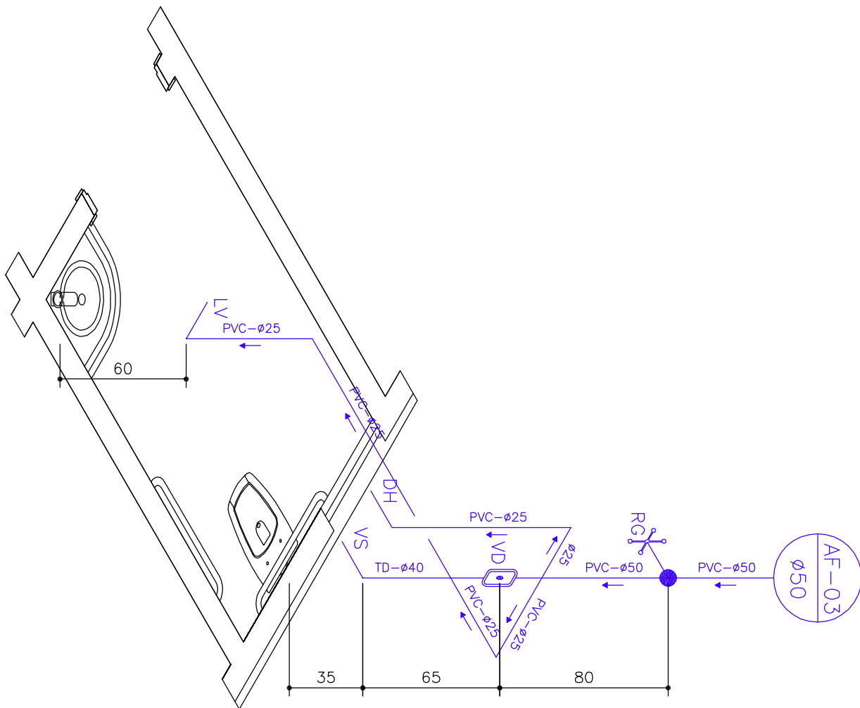
Isométrico 03: I.S. PNE Masculino Água Fria - Pavão Térreo Esc: 1:25
