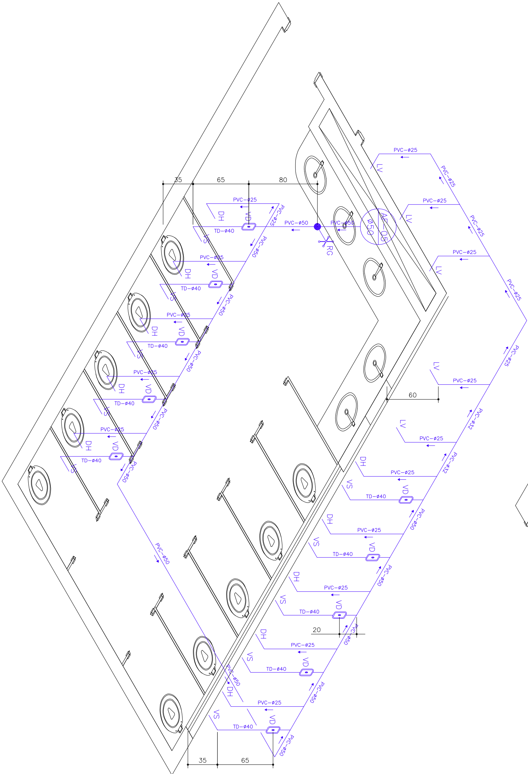
Isométrico 01: I.S. Masculino Água Fria - Pavão Térreo Esc: 1:25
