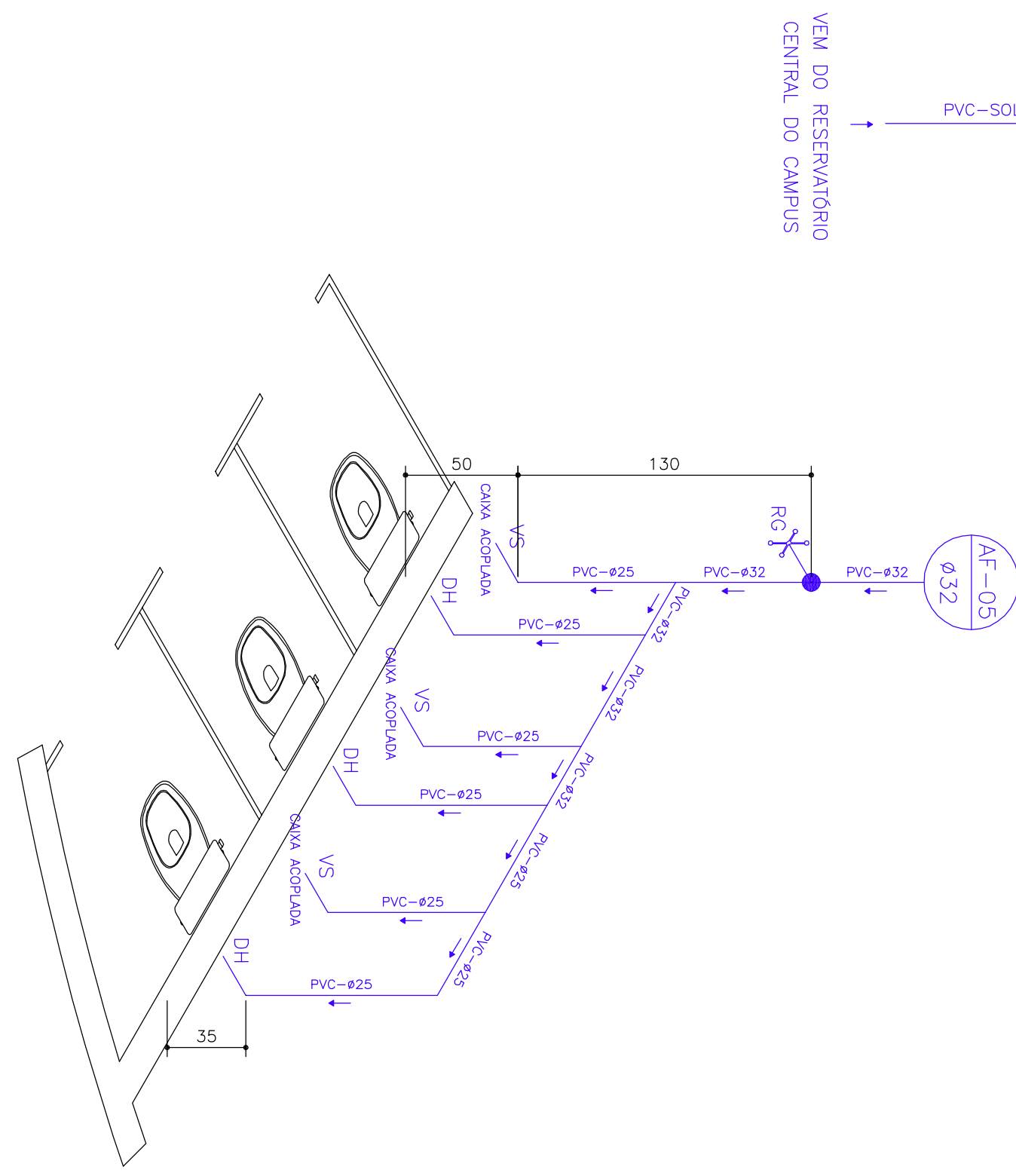
Isométrico 05: I.S. Feminino Água Fria - 1º Pavto ESC: 1:25
