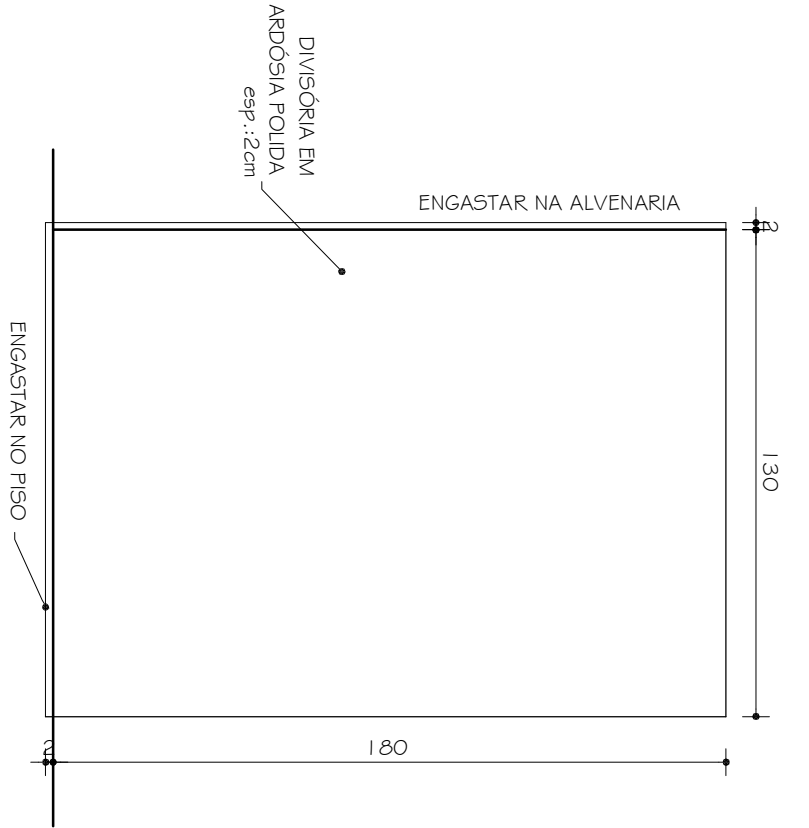
DIVISÓRIA DO1 VISTA 6 UNIDADES ESC. 1:20
