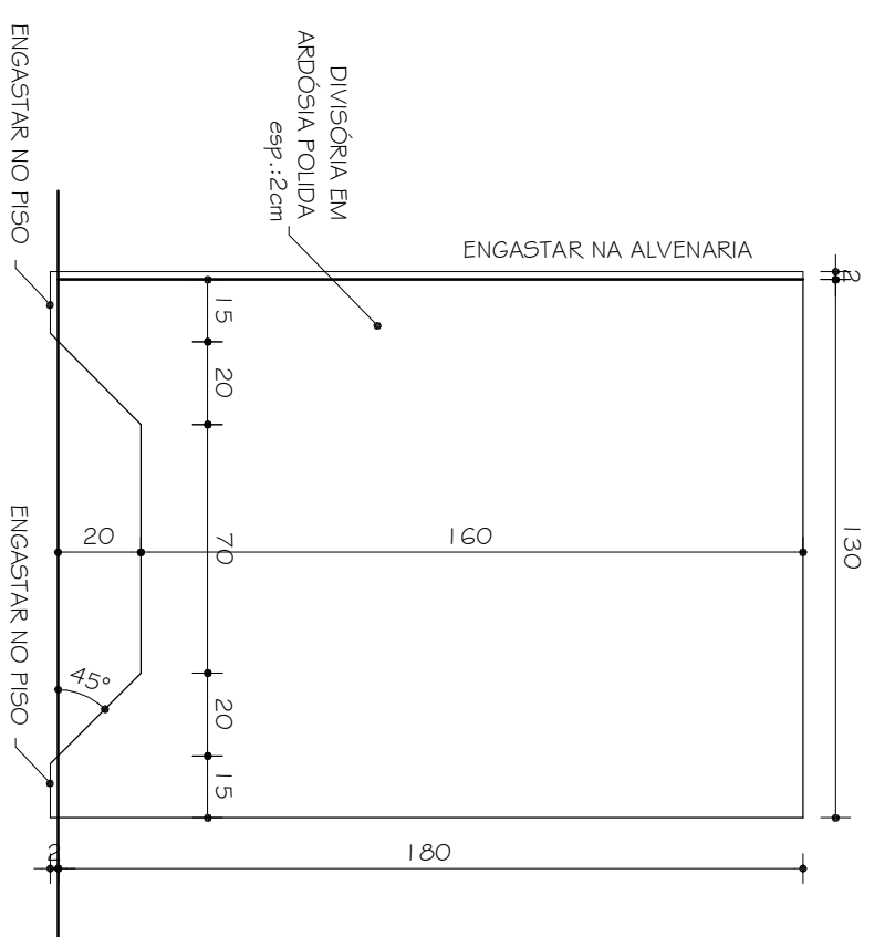
DIVISÓRIA DO6 VISTA 4 UNIDADES ESC. 1:20
