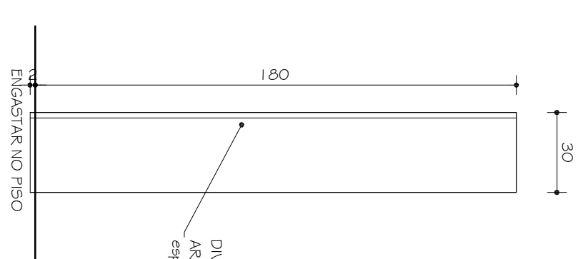
DIVISÓRIA DO3 VISTA 2 UNIDADES ESC. 1:20
