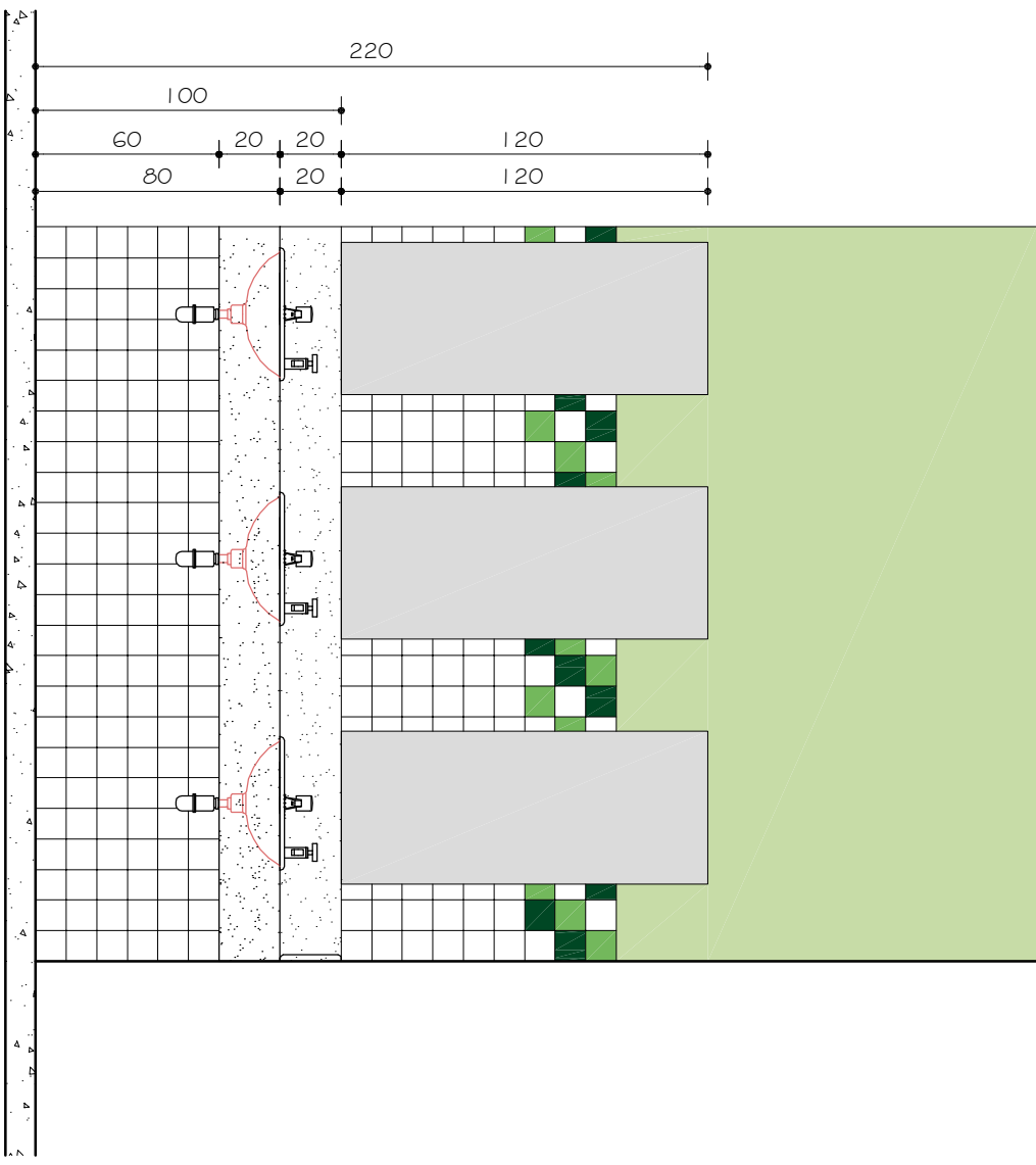
BANCA DA BOI IGUAL A BANCA DA BO2 INVERTIDA VISTA A ESC. 1:25
