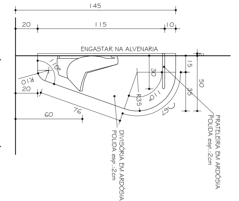
DIVISÓRIA / MICTÓRIO DO4 VISTA 4 UNIDADES ESC. 1:20
