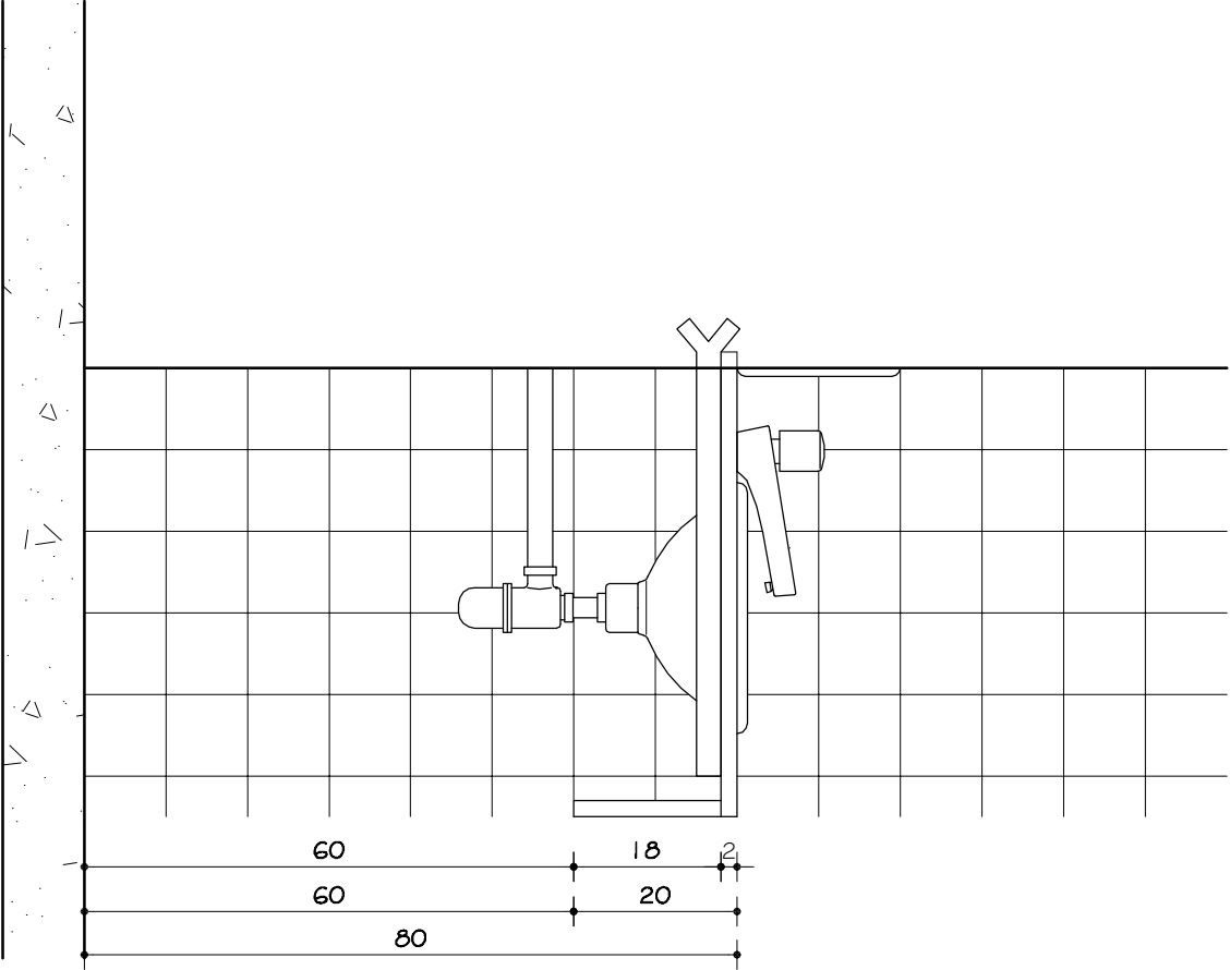
BANCA DA BOI IGUAL A BANCA DA BO2 INVERTIDA CORTE AA ESC. 1:10
