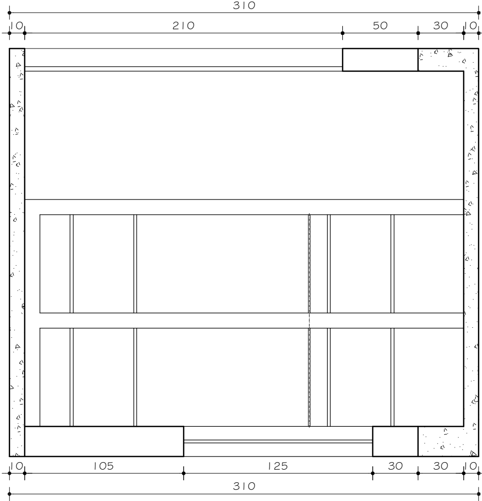
QUARTO 04 VISTA A ESC. 1:25
