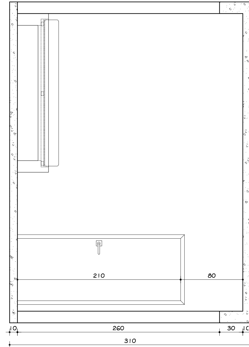
QUARTO 04 VISTA B ESC. 1:25
