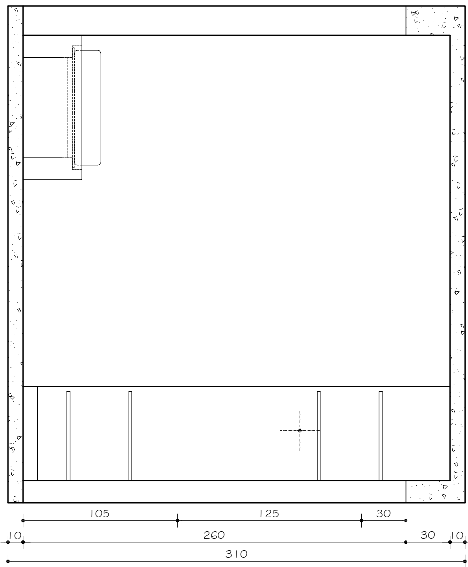
QUARTO 03 VISTA A ESC. 1:25
