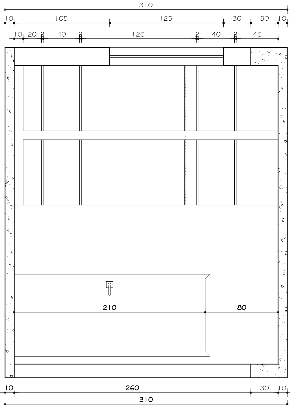
QUARTO 03 VISTA D ESC. 1:25
