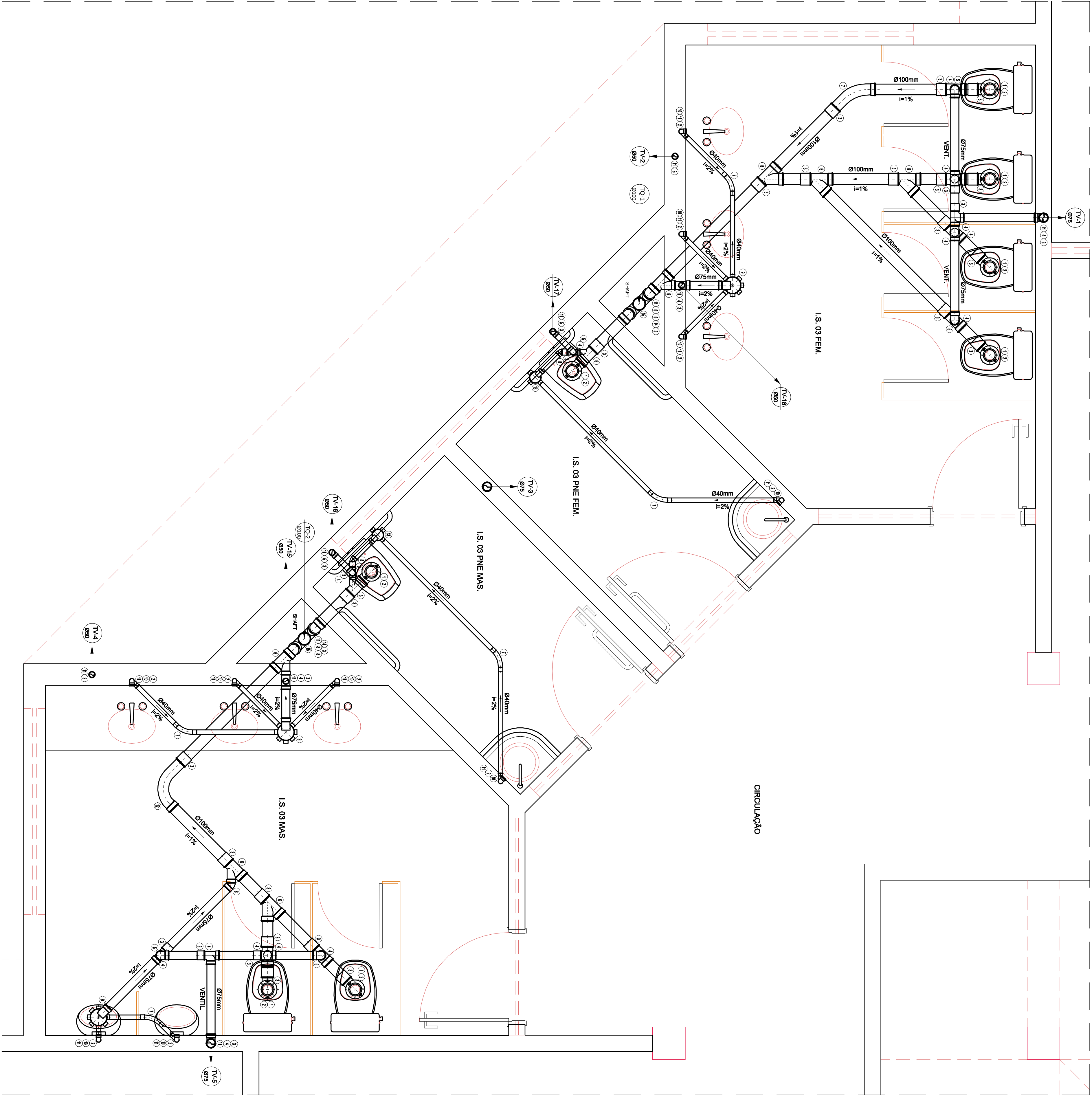
DETALHE 3 Esc. 1/20
