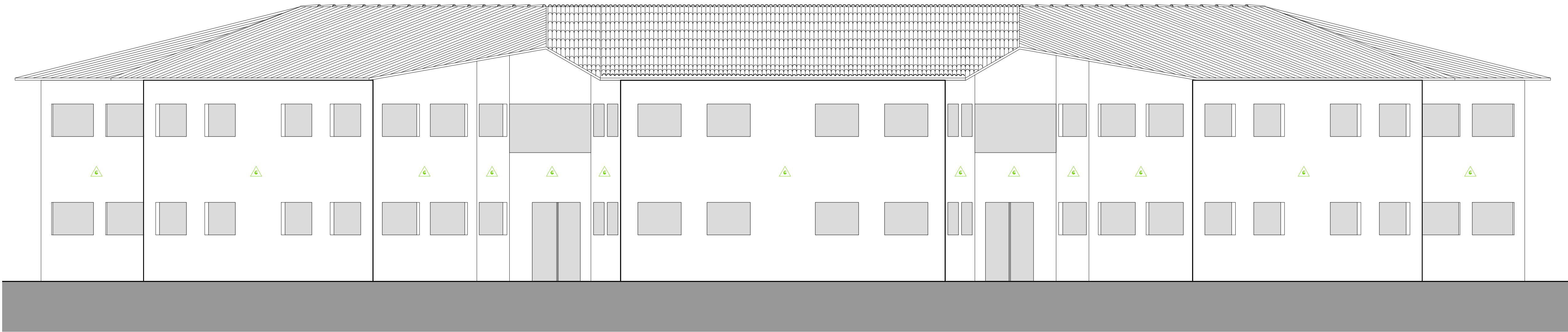
FACHADA A ESC. 1:75
