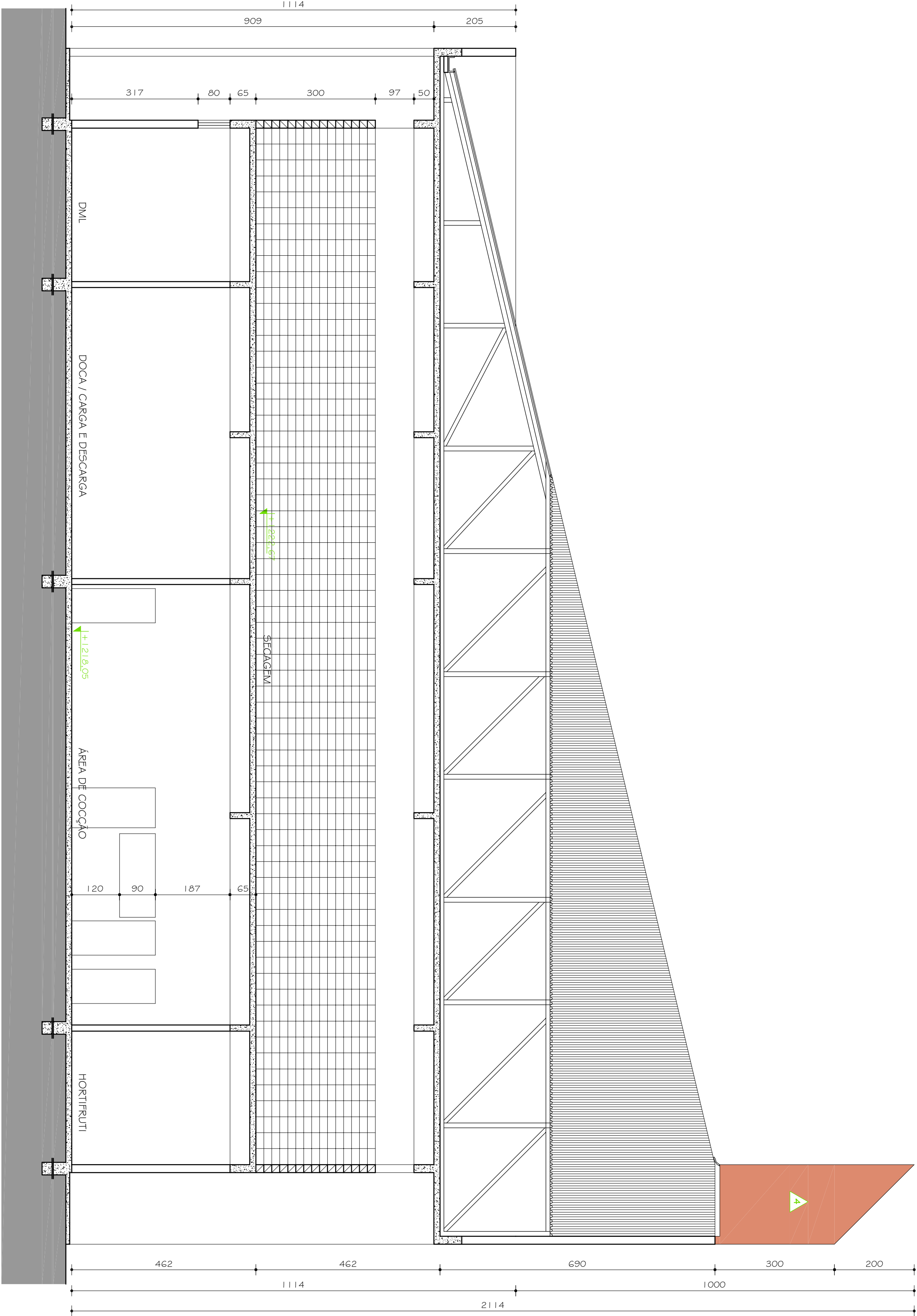
BLOCO 06 CORTE AA
