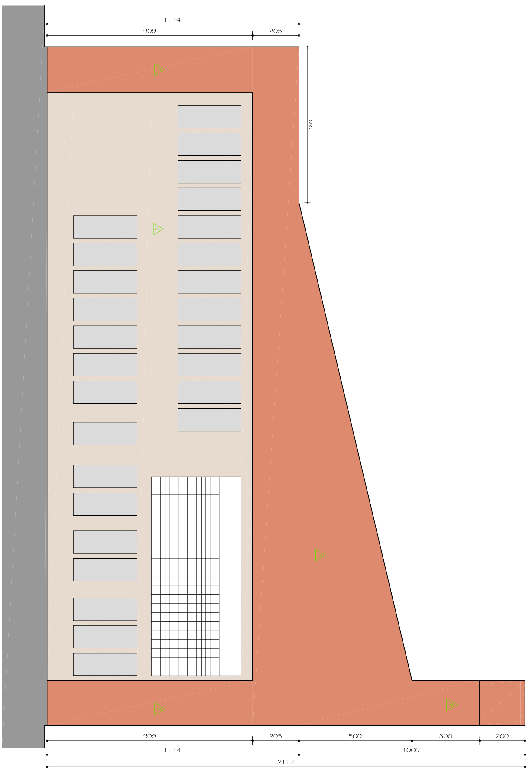
BLOCO 06 FACHADA NORDESTE ESC. 1:100
