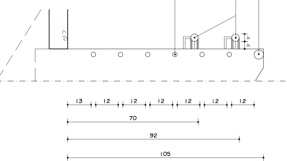
DETALHE 02 - GUARDA-CORPO ESC. 1:10
