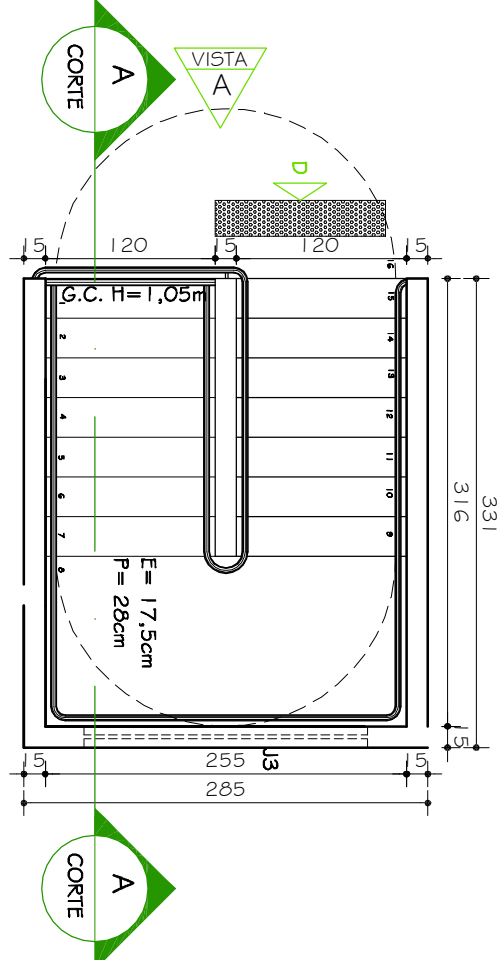
ESCADA E03 PLANTA 2º PAVIMENTO ESC. 1:50
