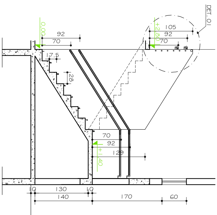
ESCADA E03 CORTE AA ESC. 1:50
