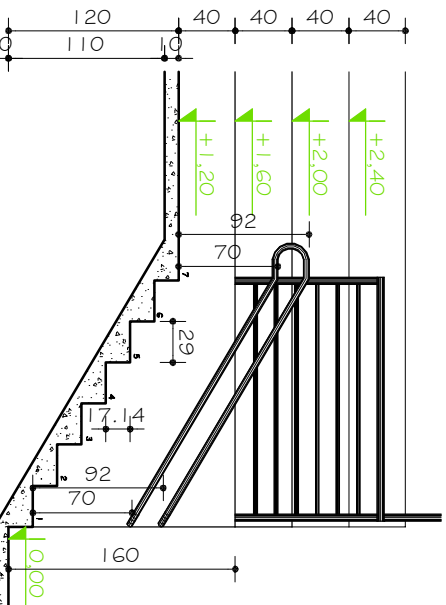
ESCADA E01 IGUAL A E02 INVERTIDA CORTE AA ESC. 1:50
