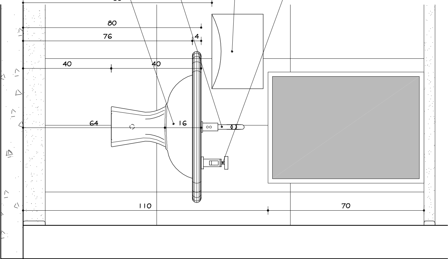
LAVATÓRIO PLANTA ESC. 1:10
