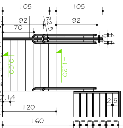
ESCADA E01 IGUAL A E02 INVERTIDA VISTA A ESC. 1:50
