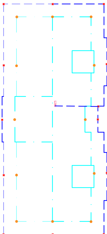
PLANTA DE COBERTURA Esc. 1:200 CASA DE APOIO
