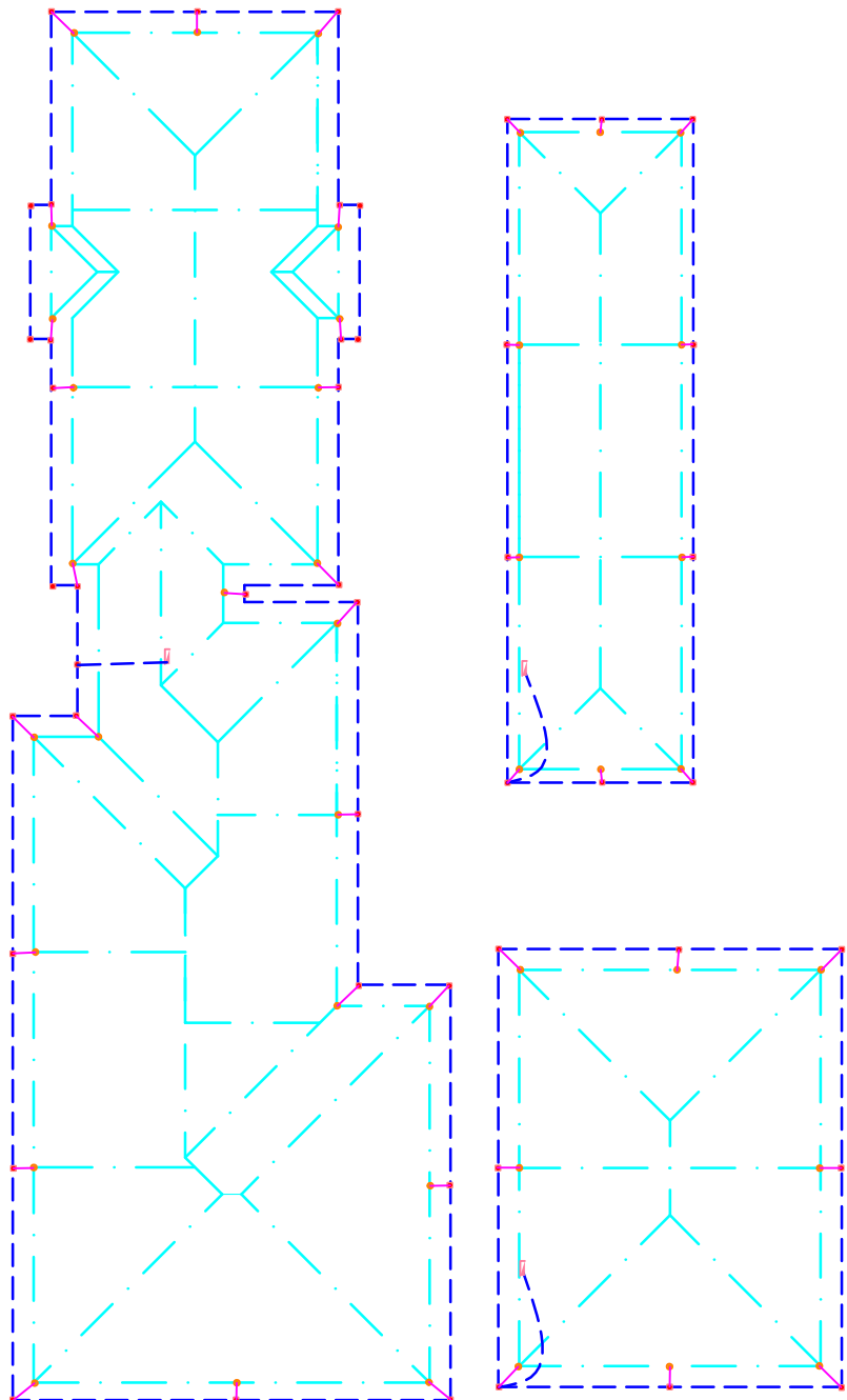
PLANTA COBERTURA Esc. 1:200 FISIOTERAPIA - 2 ANDARES
