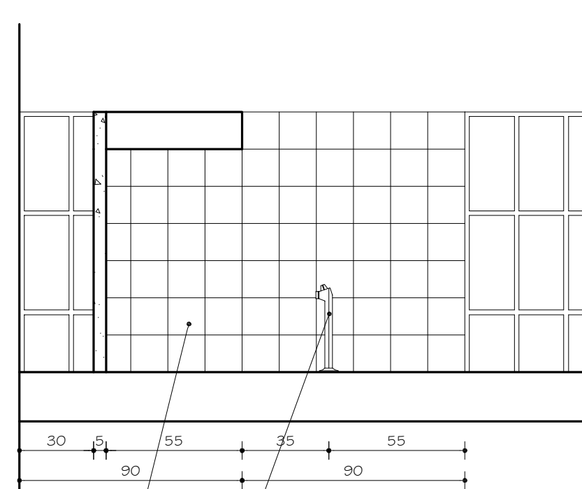
TANQUE TQ2 CORTE AA ESC. 1:20
