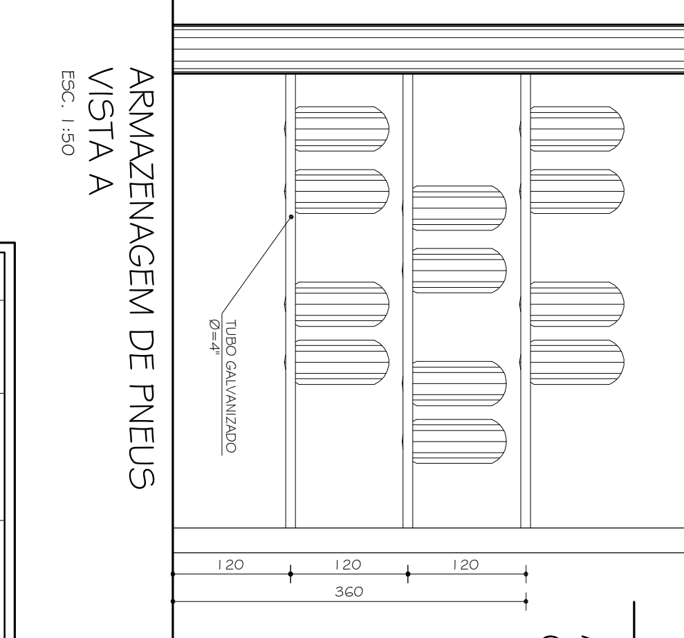
ARMAZENAGEM DE PNEUS CORTE AA ESC. 1:50
