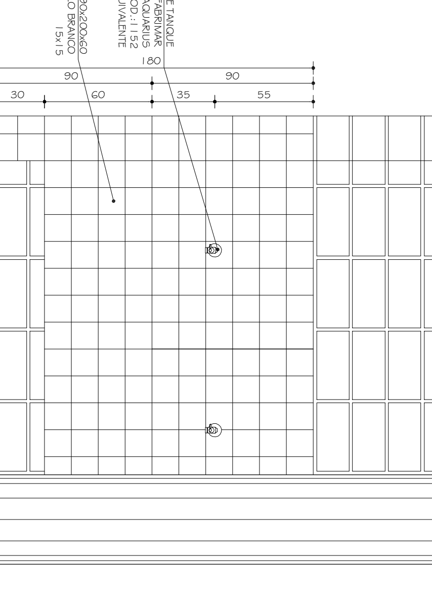
TANQUE TQ2 VISTA A ESC. 1:20
