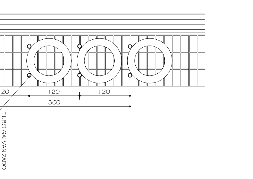
DIVISÓRIA DO6 VISTA ESC. 1:20
