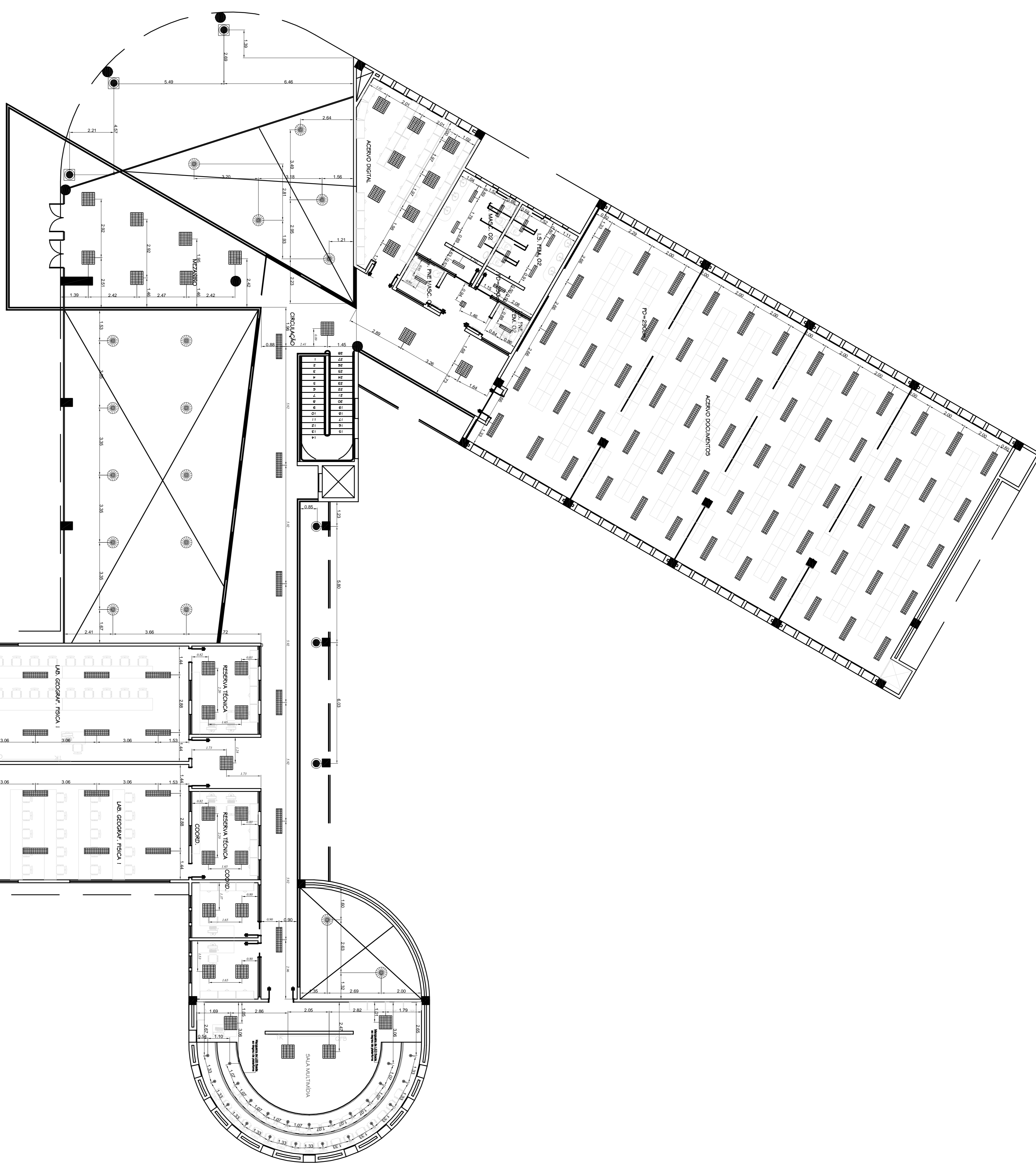
1 PONTOS ELÉTRICOS 1º PVTO ESC 1:100
