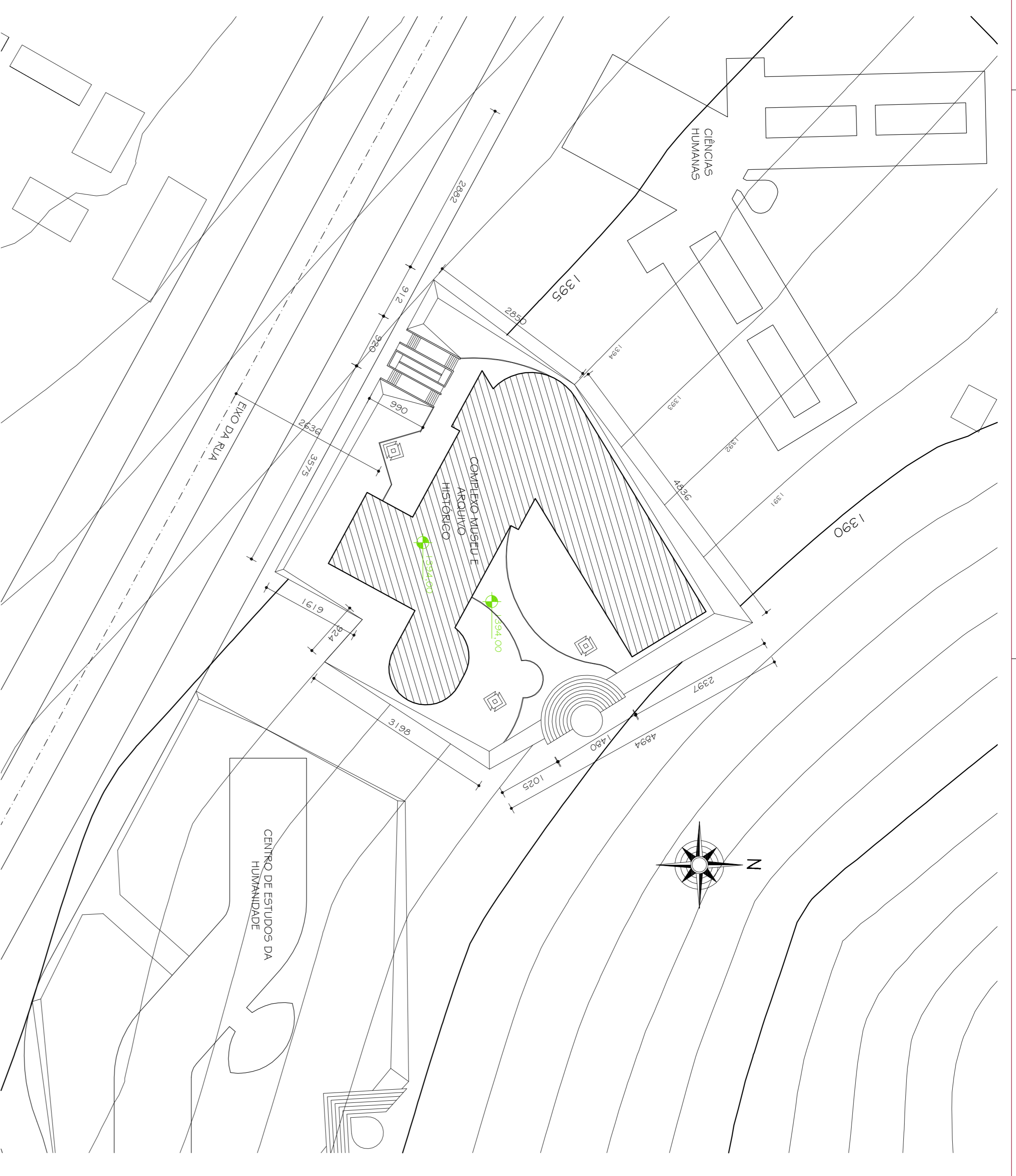
COMPLEXO MUSEU E ARQUIVO HISTÓRICO PLANTA LOCAÇÃO Esc. 1:500
