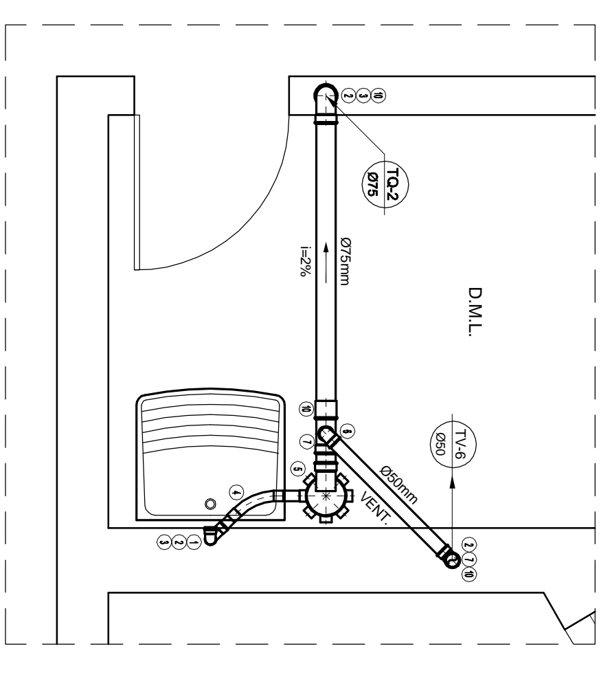
DETALHE 6 ESCALA: 1/20
