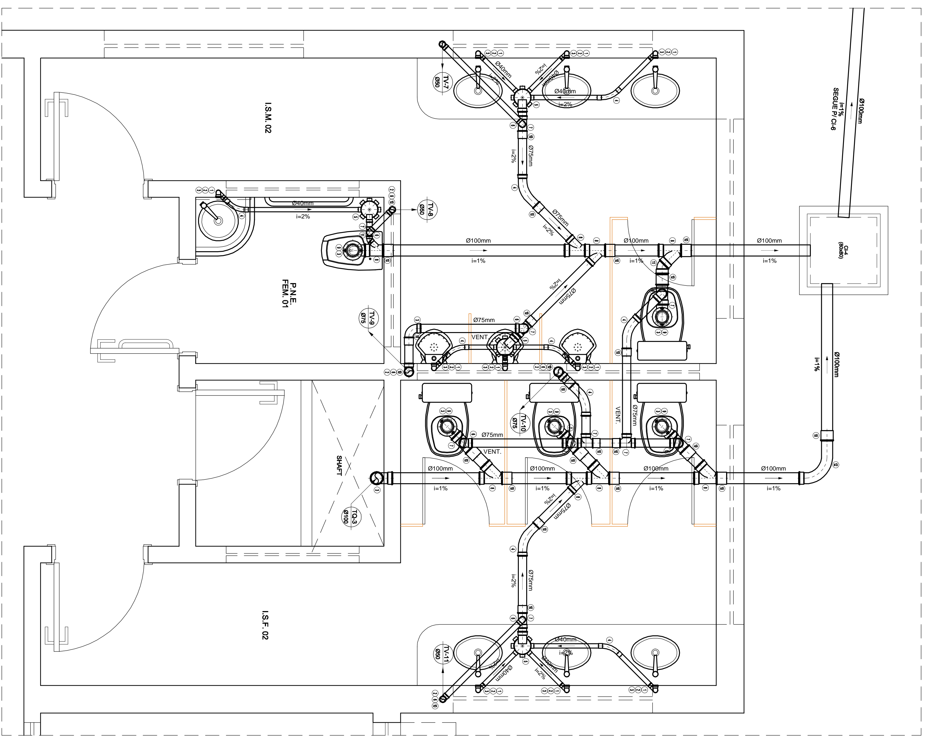
DETALHE 3 ESCALA: 1/20
