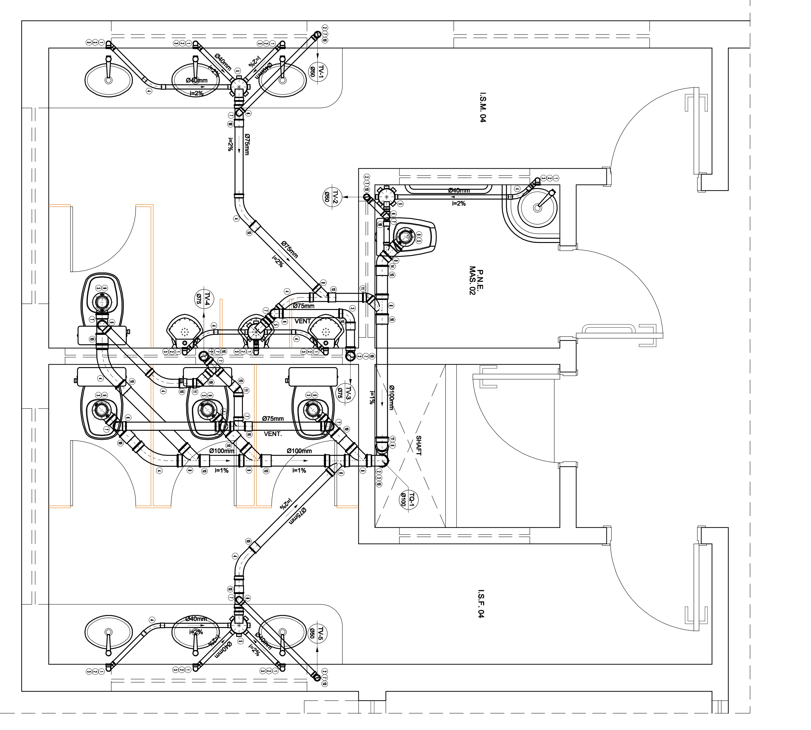
DETALHE 5 ESCALA: 1/20
