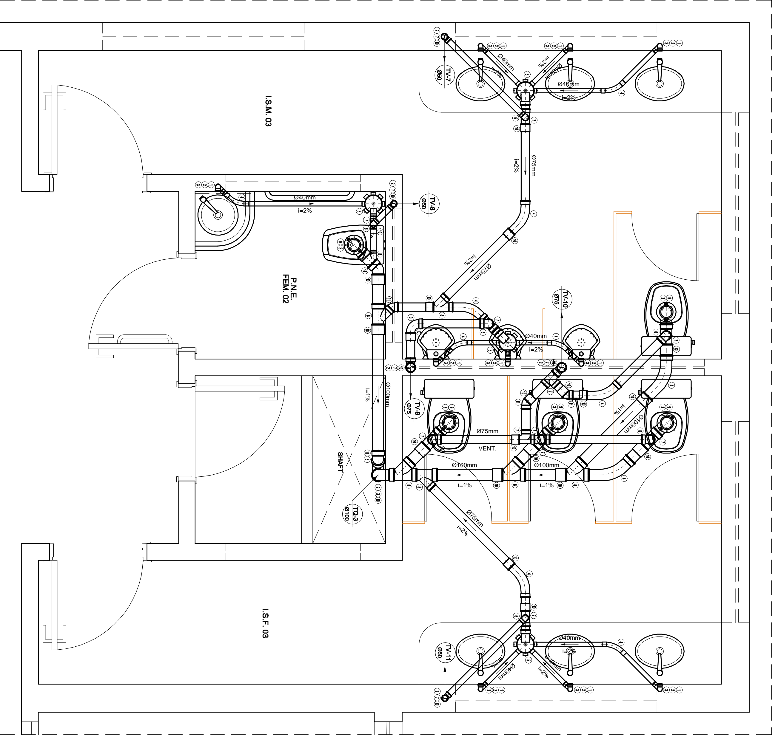
DETALHE 7 ESCALA: 1/20
