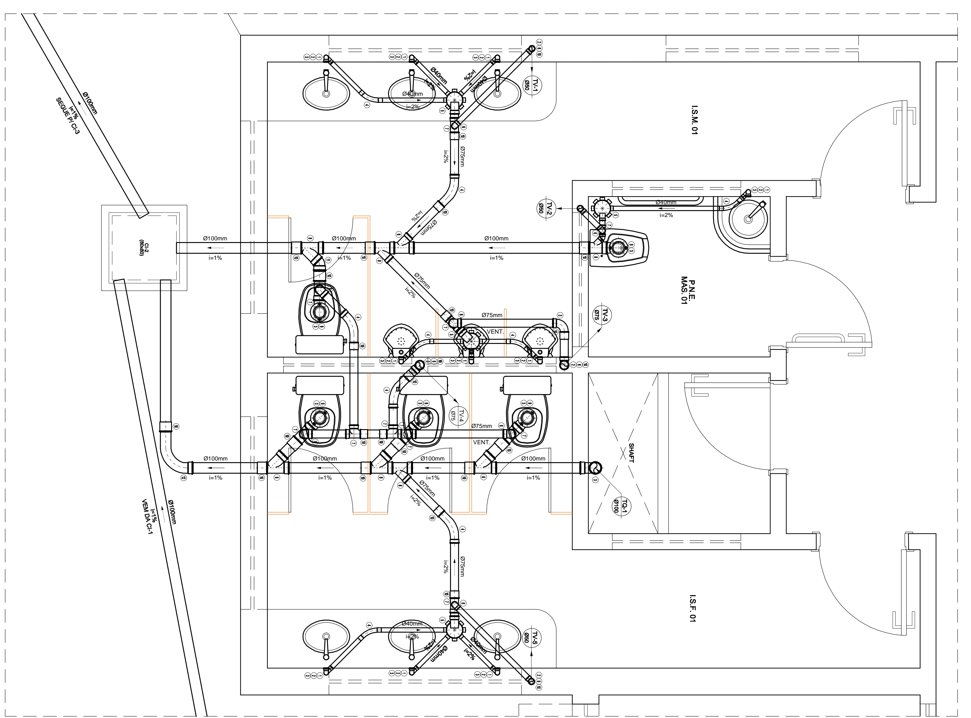
DETALHE 1 ESCALA: 1/20
