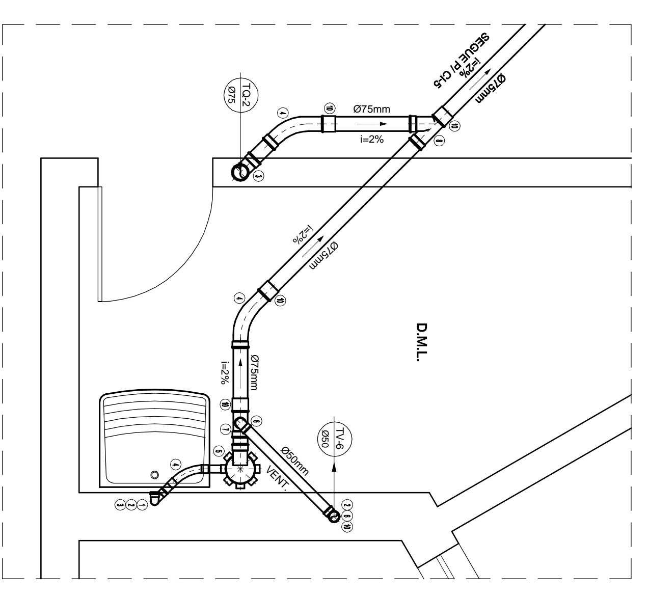
DETALHE 2 ESCALA: 1/20
