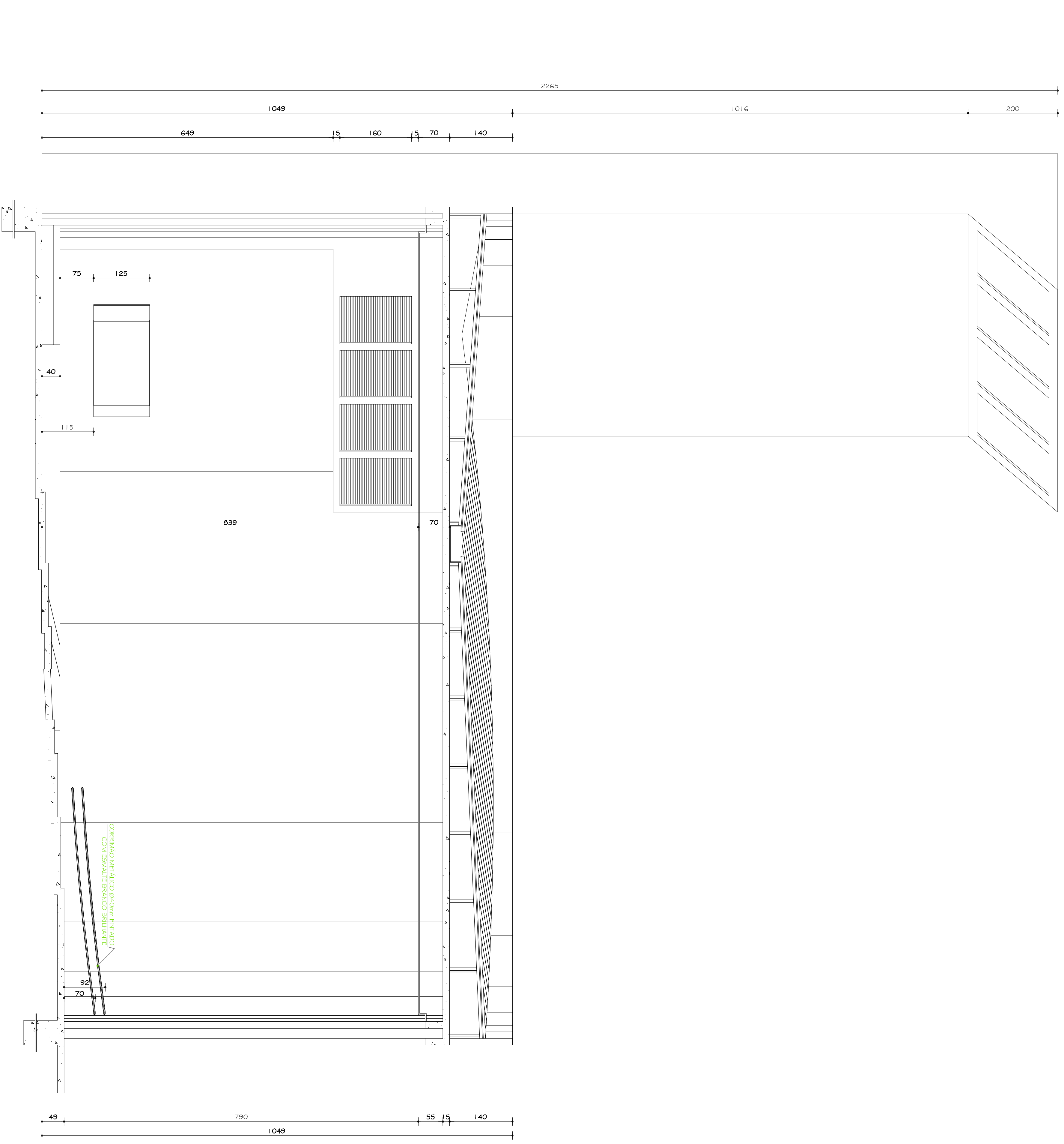
DETALHE AUDITÓRIO CORTE AA Esc. 1:50
