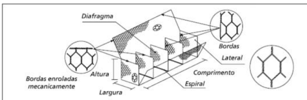
Figura 1 – Elementos constituintes dos gabiões tipo caixa.
