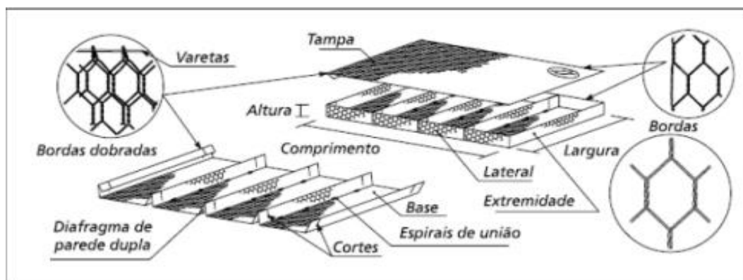
Figura 2 – Elementos constituintes do gabião tipo colchão reno.
