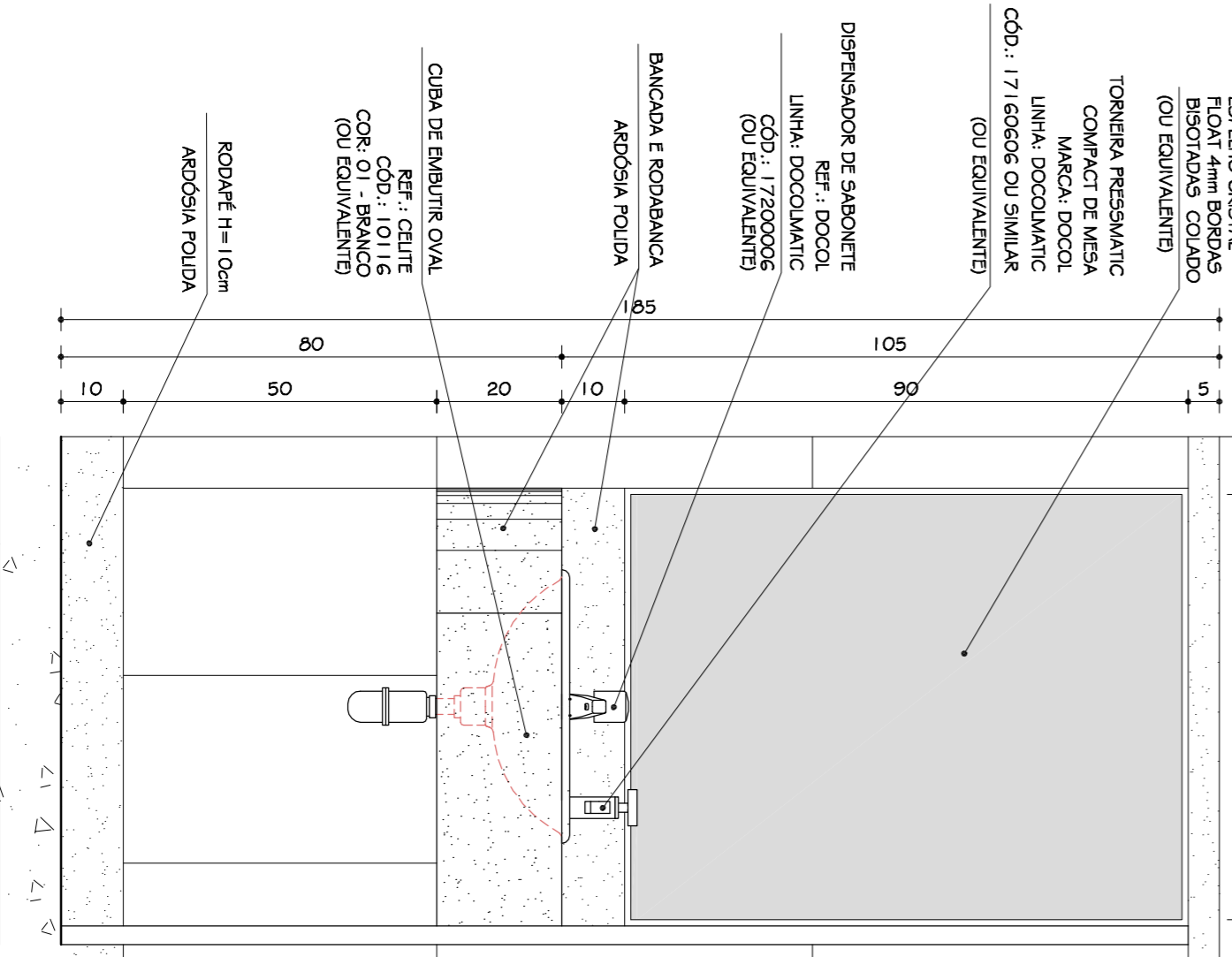
B02 - BANCADA VESTIÁRIO ÁRTIBROS VISTA A ESC. 1:10
