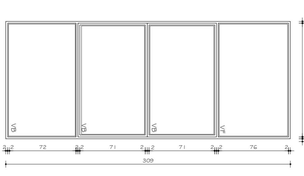
JO5 VISTA ESC. 1:25
